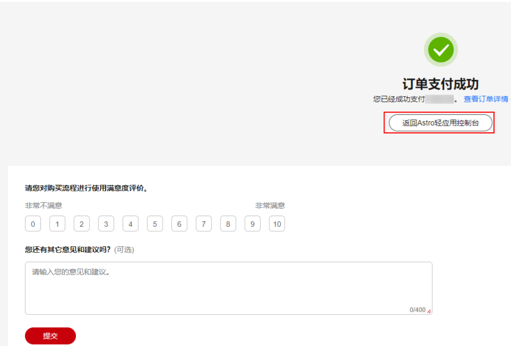
图 1-5 返回控制台
