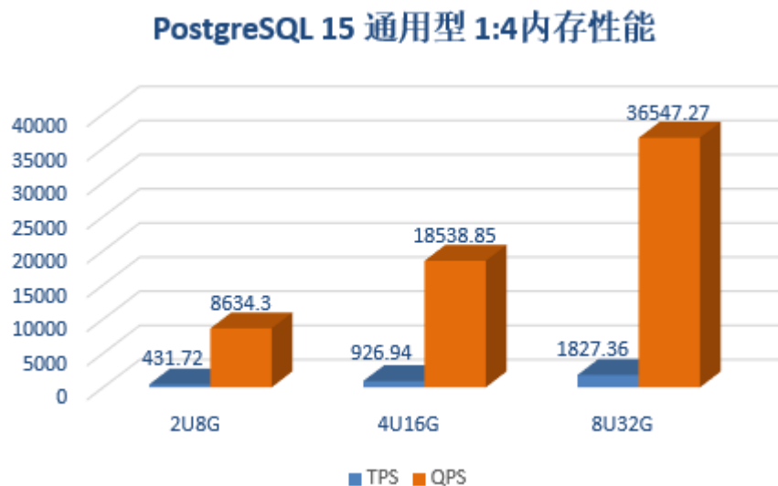
图 5-2 CPU:内存=1:4
