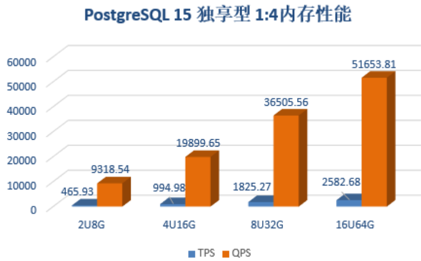
图 5-4 CPU:内存=1:4
