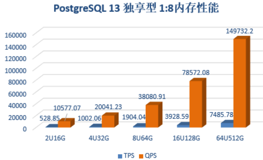
图 3-4 CPU:内存=1:8
