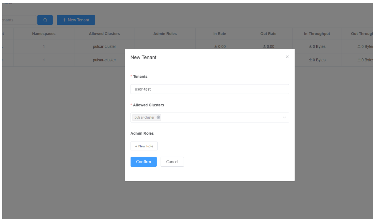
图 3-29 添加新租户
