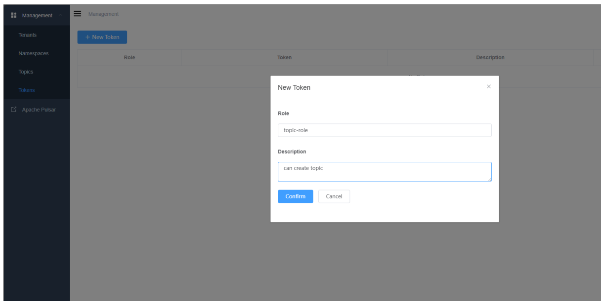
图 3-32 生成 token
