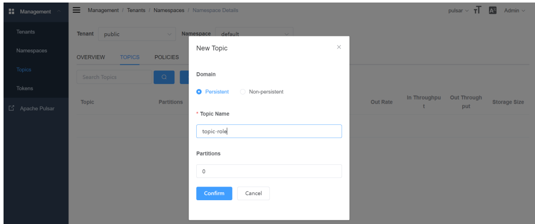
图 3-31 添加 topic
