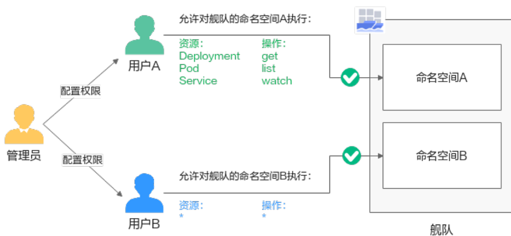
图 7-1 Kubernetes 资源授权示意图
