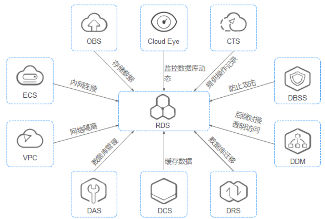
图 10-1 RDS for MySQL 与其他服务的关系示意图
