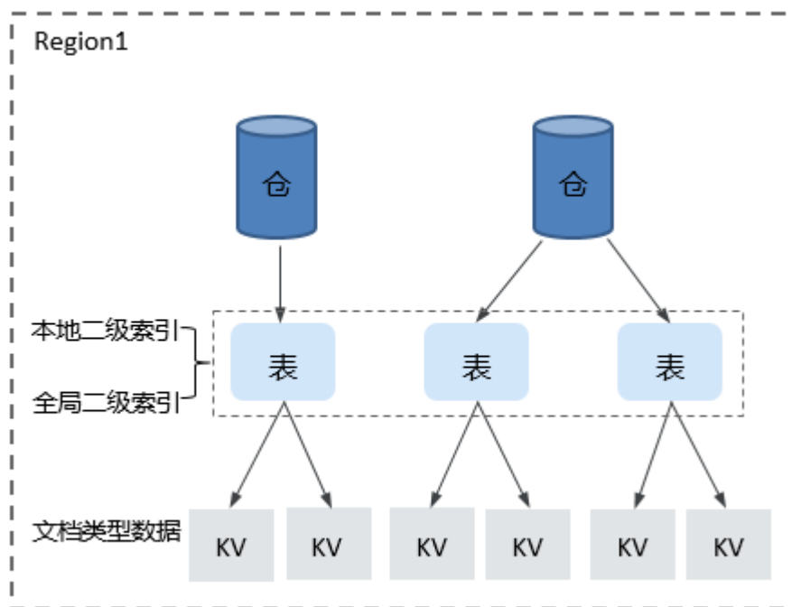
图 8-1 KVS 基本概念之间的关系
