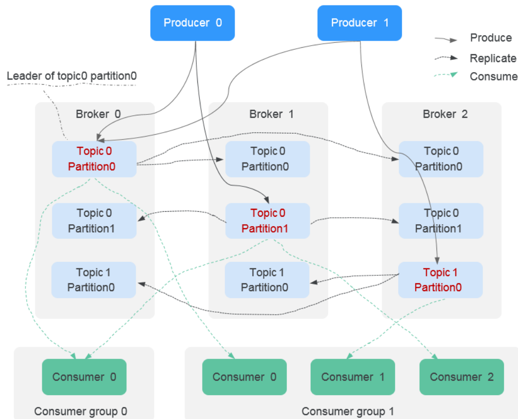
图 11-1 Kafka 消息流
