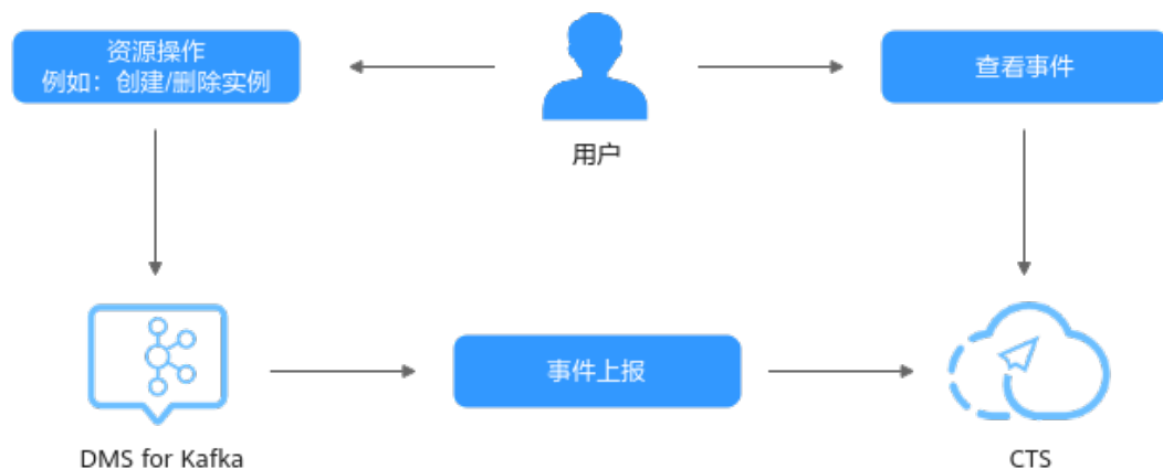
图 8-2 云审计服务
