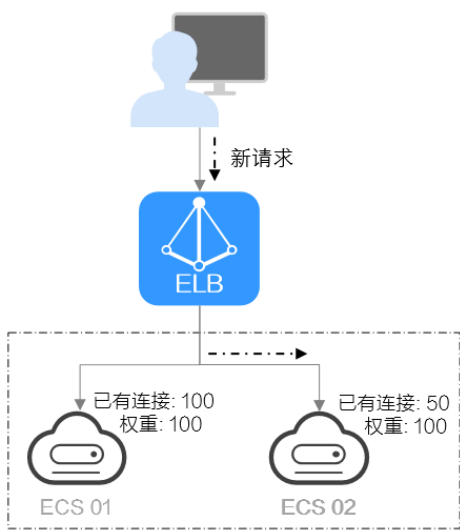
图 3-3 加权最少连接算法流量分发
