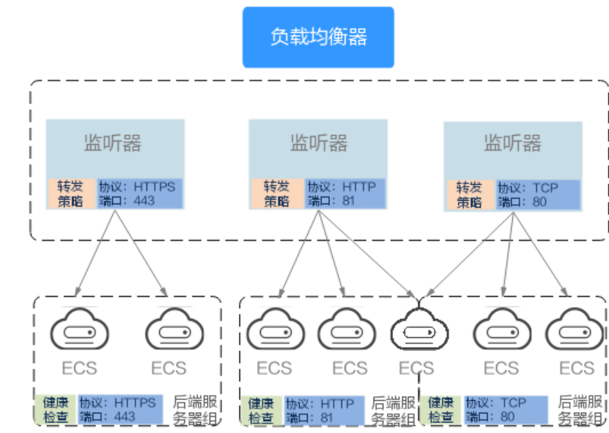
图 1-2 弹性负载均衡组件图
