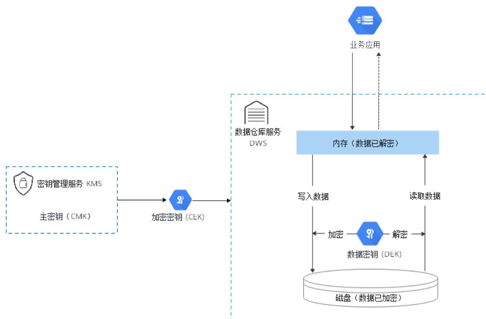
图 9-3 TDE 加解密原理
