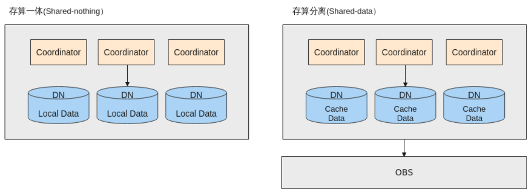
图 1-3 架构选择
