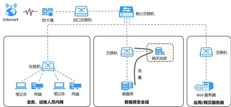
图 4-2 组网方式
