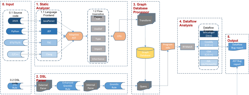
图 2-1 DSL 引擎工作原理
