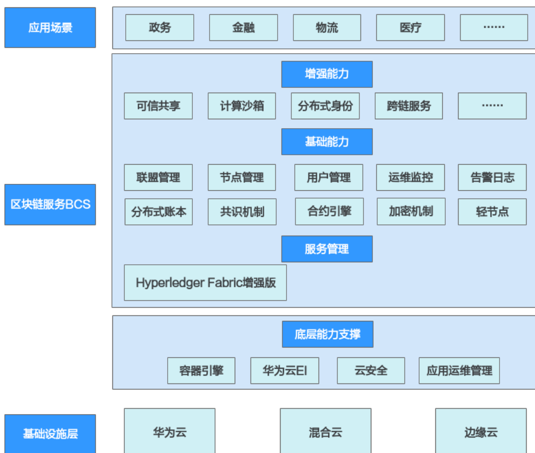
图 2-1 产品架构
