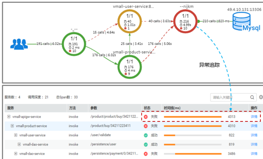
图 2-2 调用链追踪
