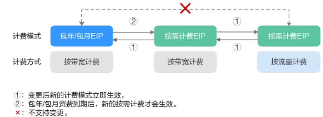
图 4-1 EIP 计费模式变更
