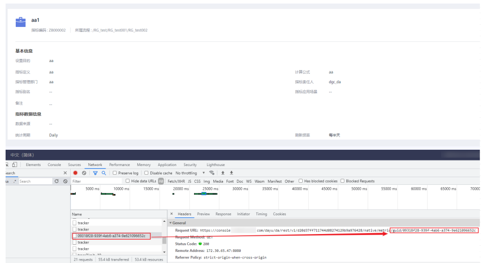
图 6-6 获取 guid
