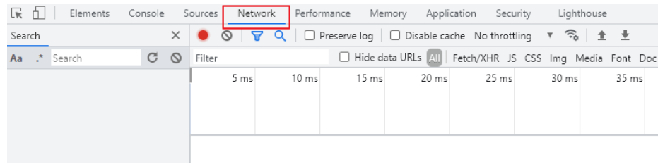
图 6-4 选择 Network
