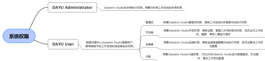
图 5-3 权限体系
