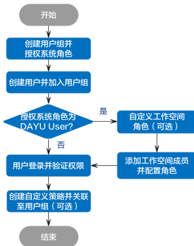
图 5-2 授权流程
