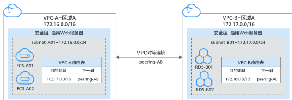
图 1-4 对等连接组网示意图
