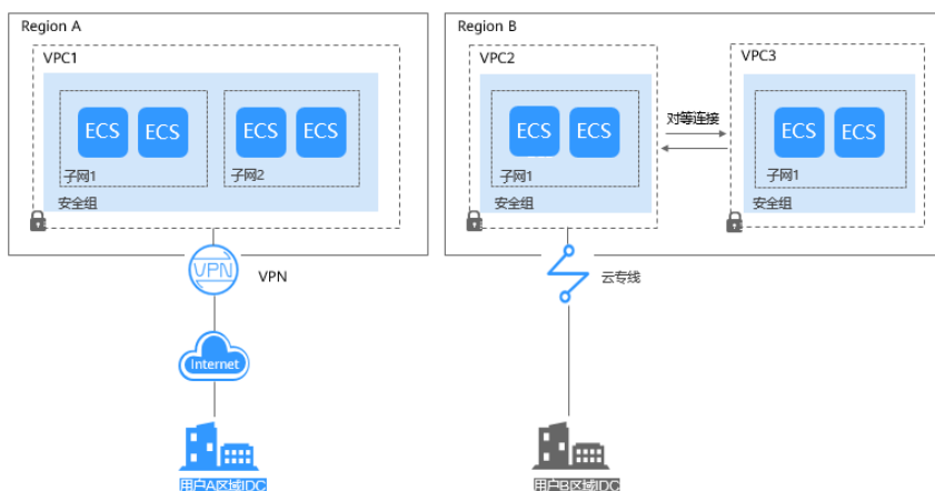
图 3-1 IDC 连接
