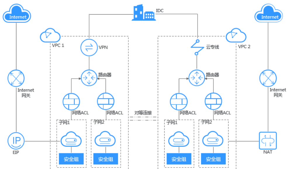
图 1-1 VPC 组成
