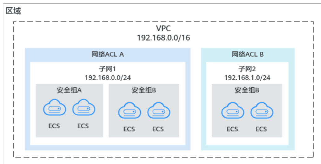
图 1-5 安全组与网络ACL
