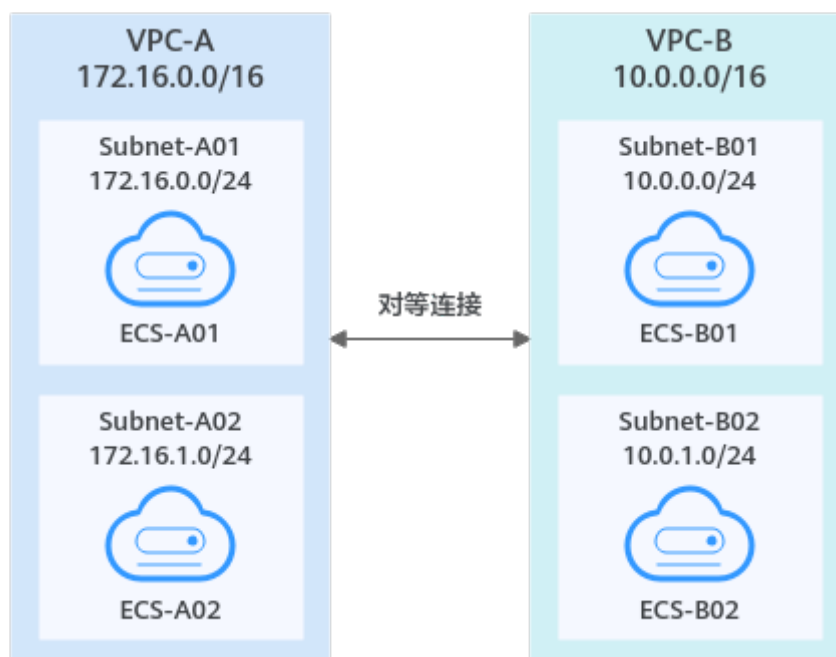
图 7-4 相互对等的两个 VPC(IPv4)
