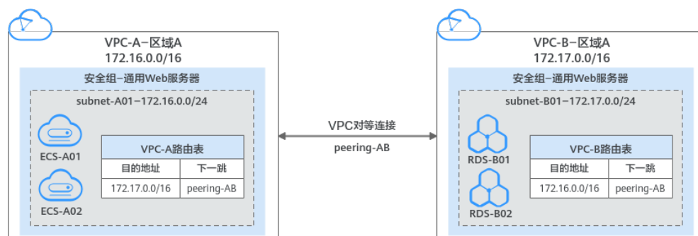
图 7-1 对等连接组网示意图
