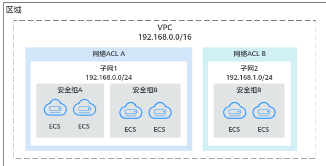
图 6-5 安全组与网络 ACL
