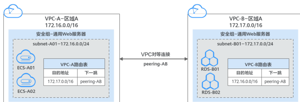
图 13-3 对等连接组网示意图
