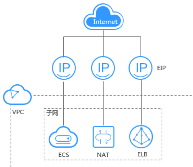
图 1-3 通过 EIP 访问公网
