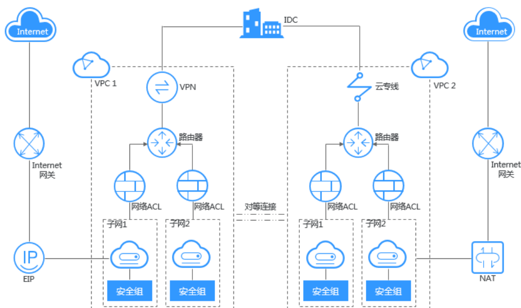
图 13-1 产品架构
