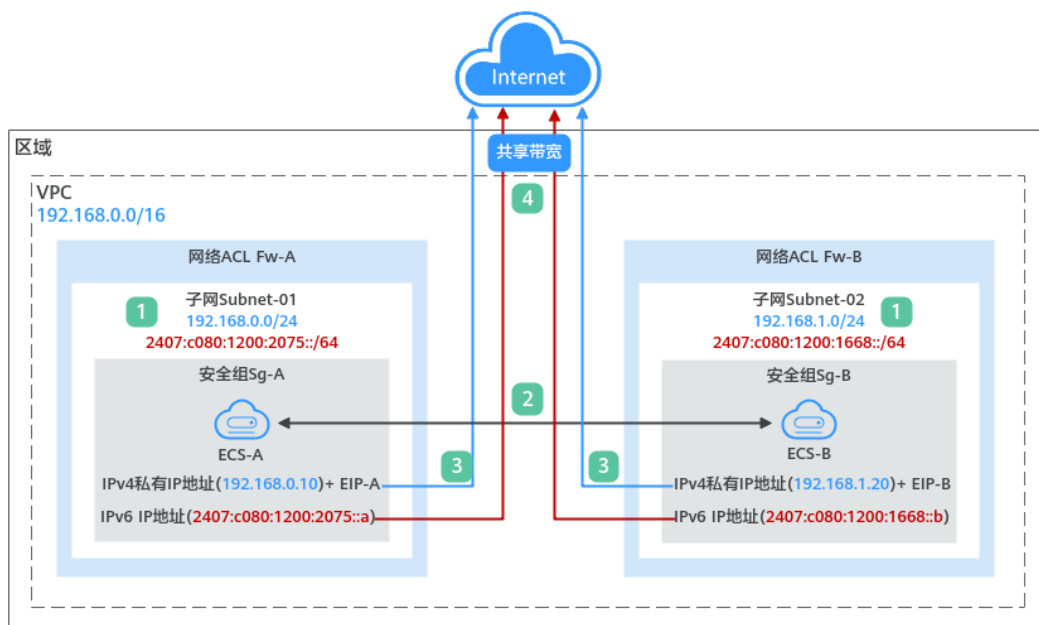
图 3-4 IPv6 双栈网络架构图(VPC/EIP)
