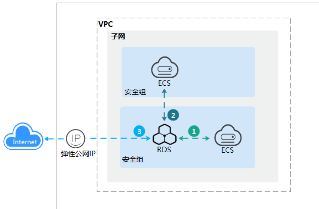
图 3-2 实例内网和公网连接
