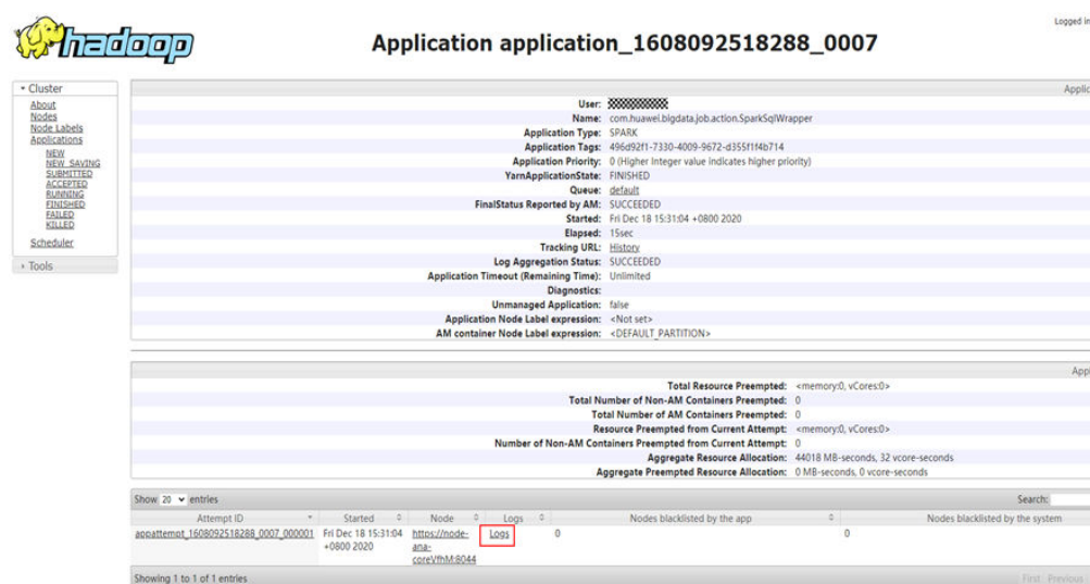
图 16-11 任务日志
