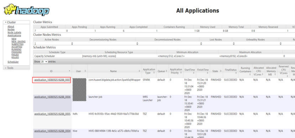
图 16-10 Yarn 的 Applications
