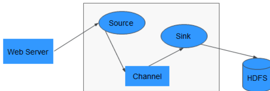
图 1-28 Flume-NG 架构
