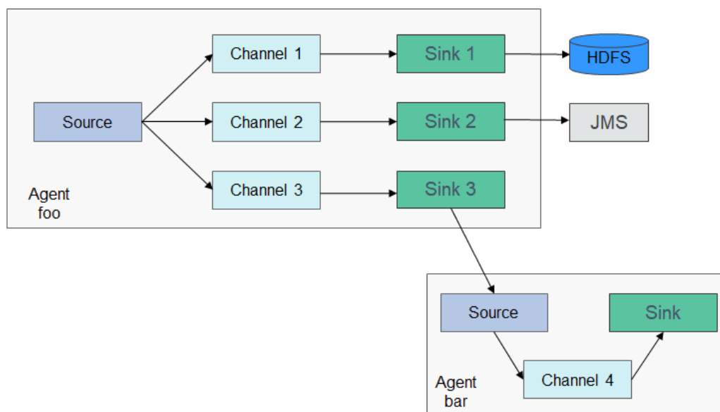
图 1-29 Flume 结构图
