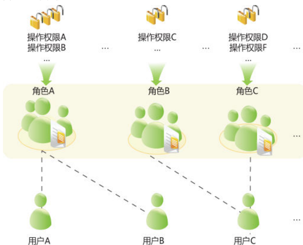
图 10-21 权限模型
