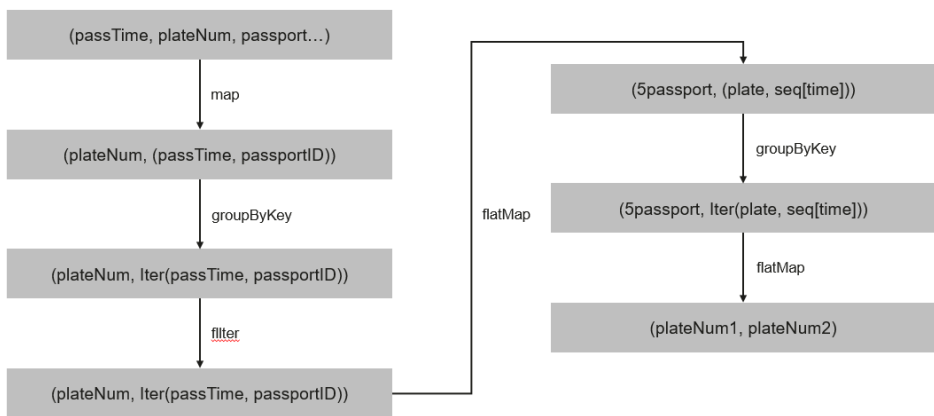
图 12-56 实现 2 逻辑
