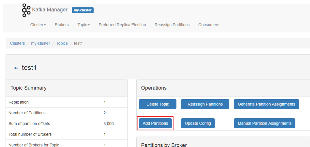
图 12-31 添加分区
