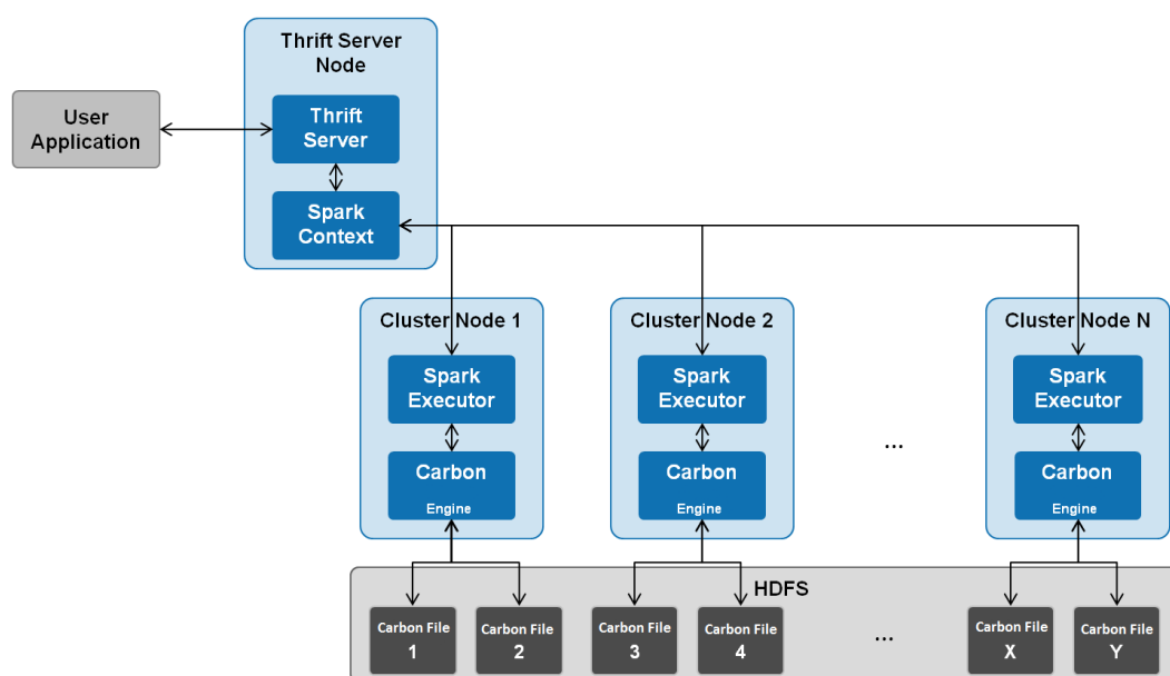
图 12-3 CarbonData 结构
