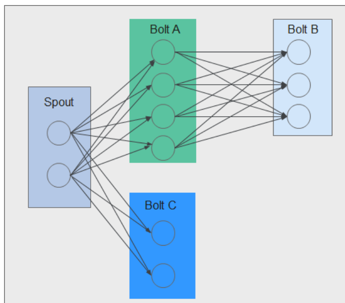
图 1-127 Topology 示意图
