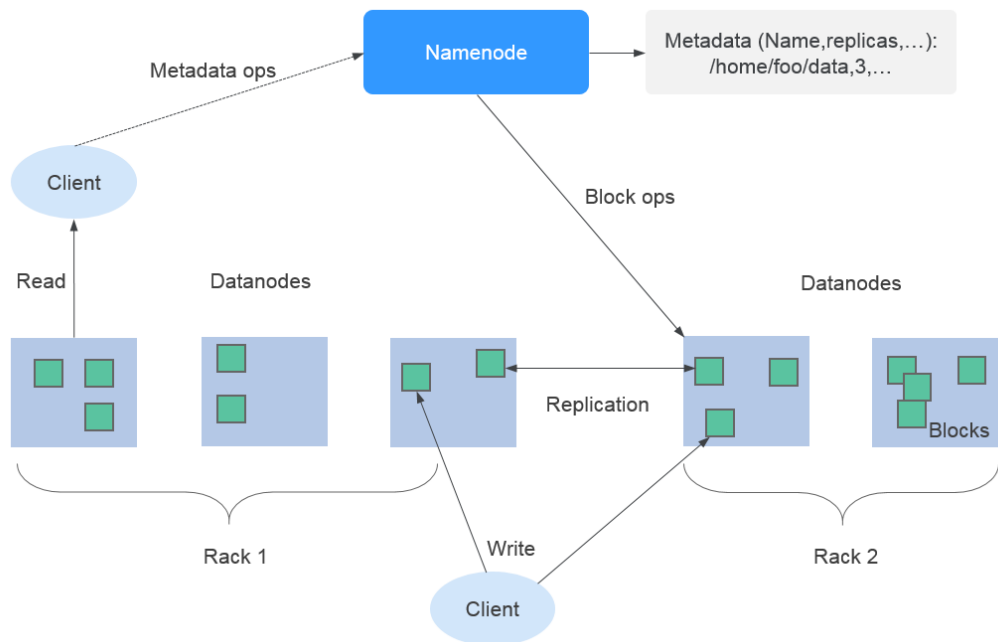
图 1-45 HDFS 架构
