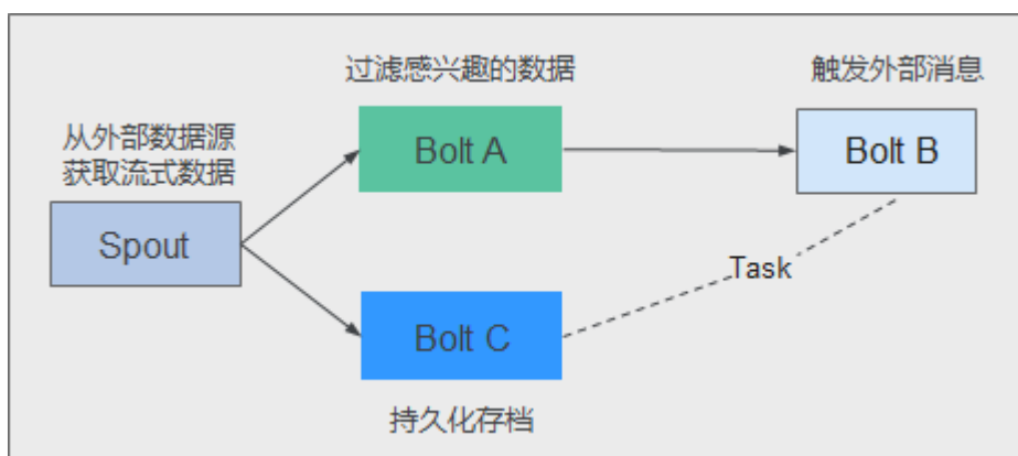
图 1-126 Topology
