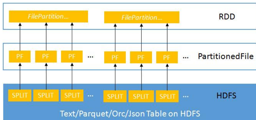
图 12-57 小文件合并
