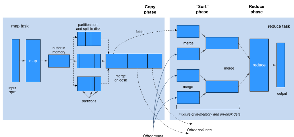
图 12-36 Shuffle 过程
