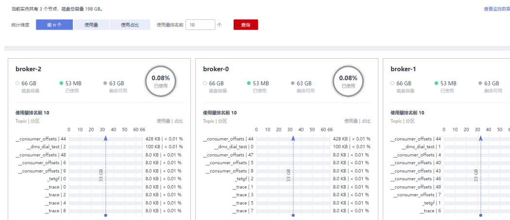
图 11-1 查看磁盘的使用量
