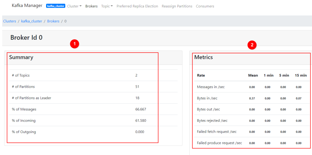
图 11-4 具体 Broker 信息
