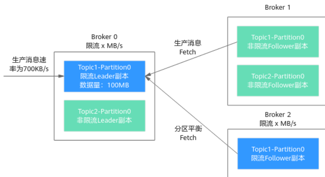
图 6-19 场景三分区平衡图
