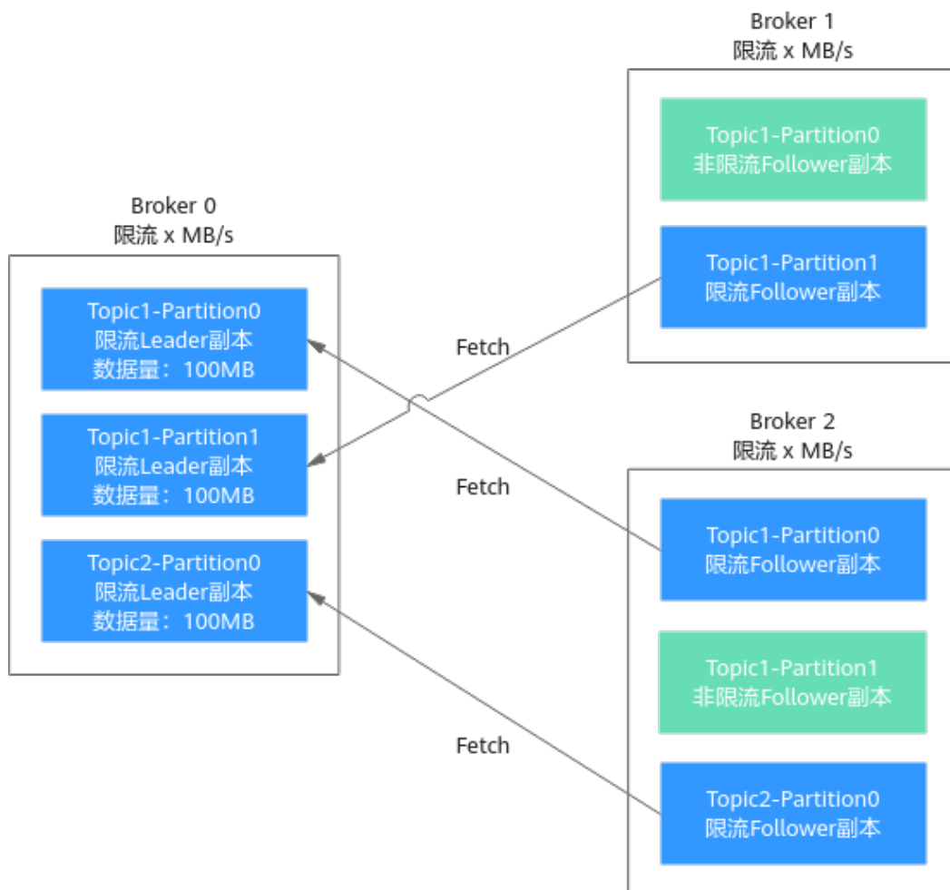
图 6-17 场景一分区平衡图
