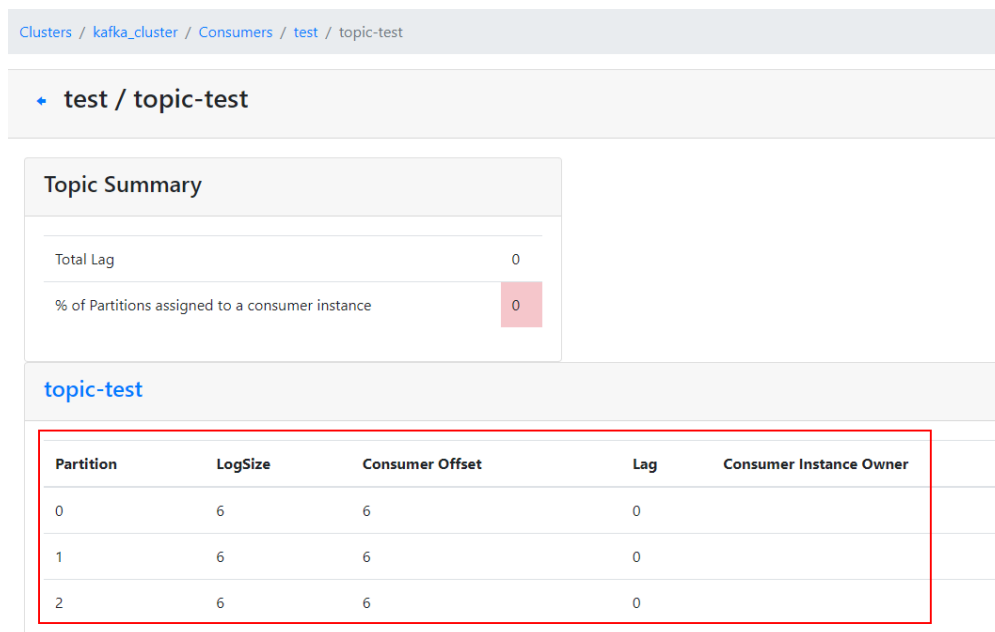
图 11-9 消费组队列详情页面
