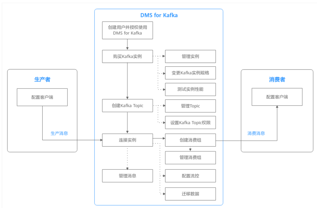
图 3-1 Kafka 业务使用流程
