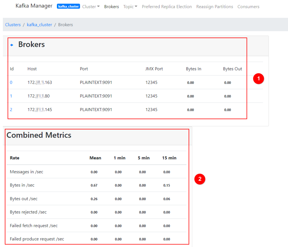
图 11-3 所有代理统计页
