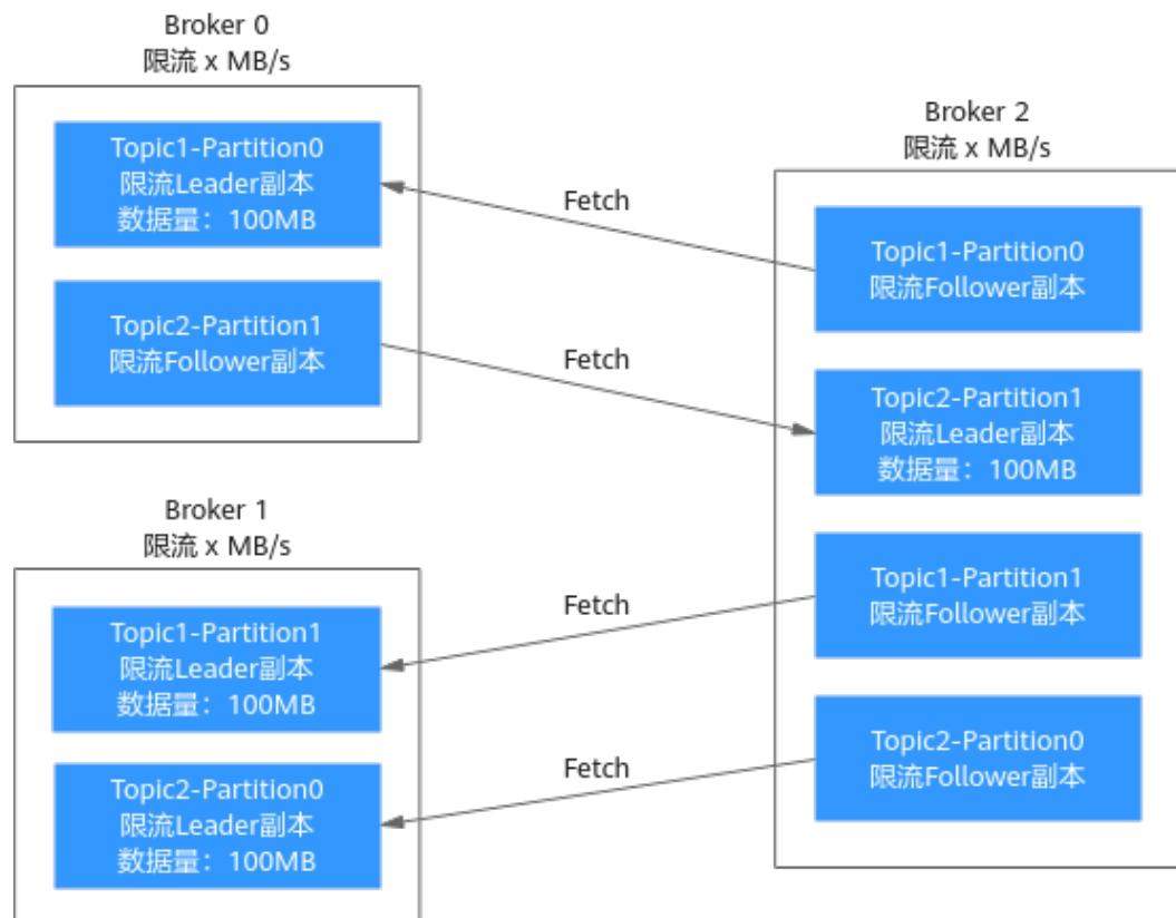
图 6-18 场景二分区平衡图
