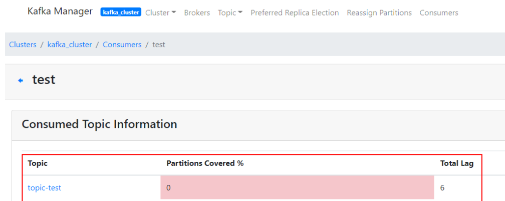
图 11-8 消费组详情页面
