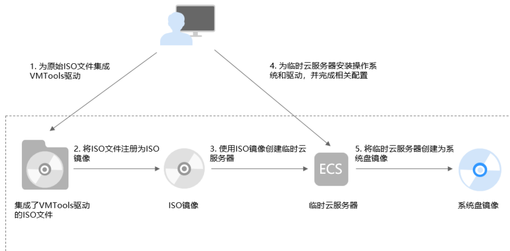
图 2-14 创建过程（Windows 系统盘镜像）
