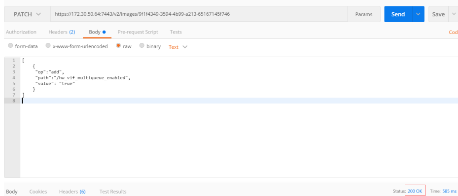
图 7-10 支持网卡多队列修改样例
