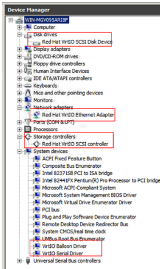
图 2-37 查看设备管理器
