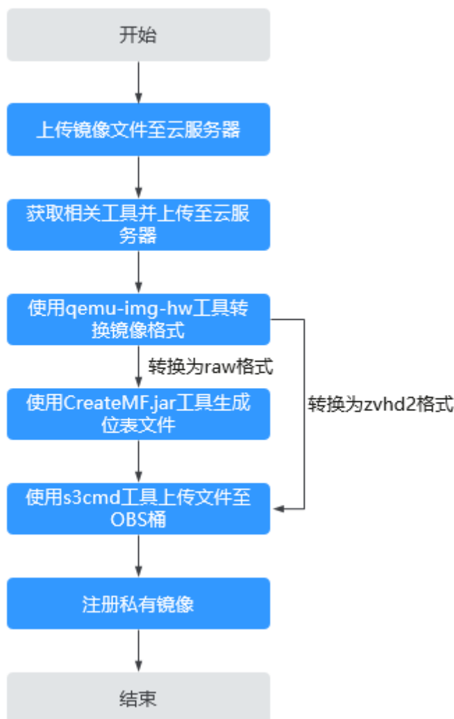
图 2-49 导入流程（基于 Linux 操作系统环境）
