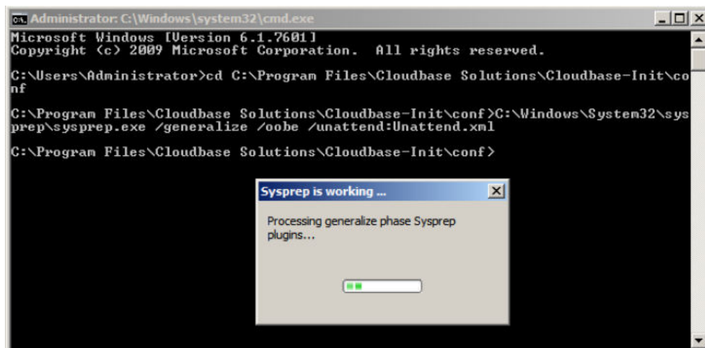
图 4-8 执行 Sysprep 操作
