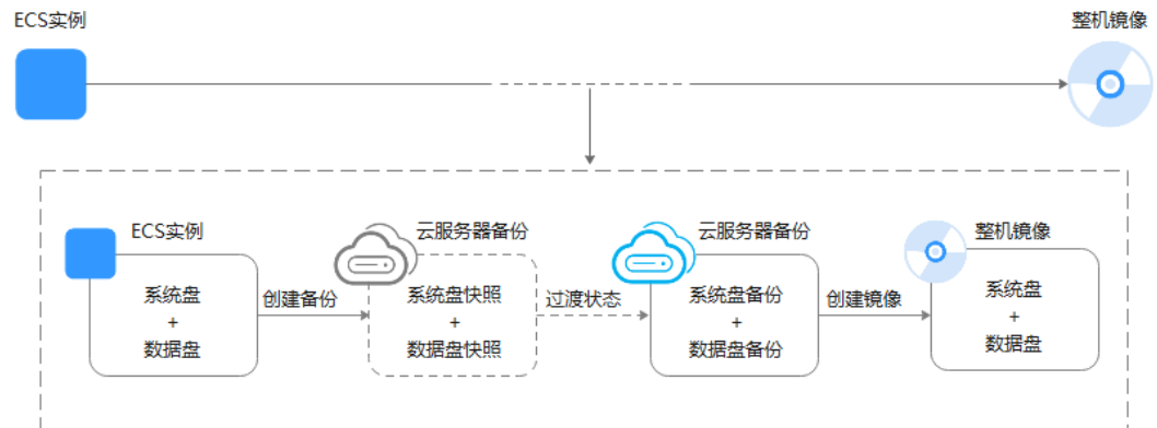
图 2-10 整机镜像创建流程
