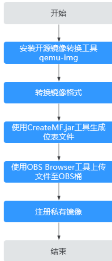
图 2-50 导入流程（基于 Windows 操作系统环境）
