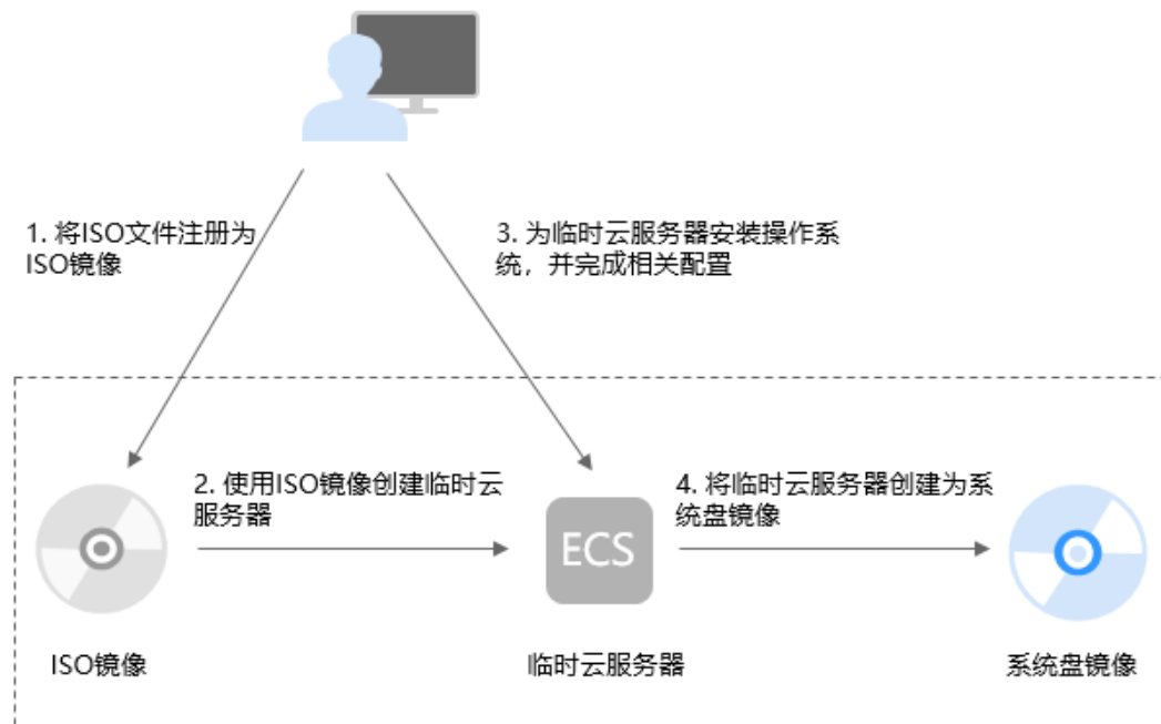
图 2-38 创建过程（Linux 系统盘镜像）
