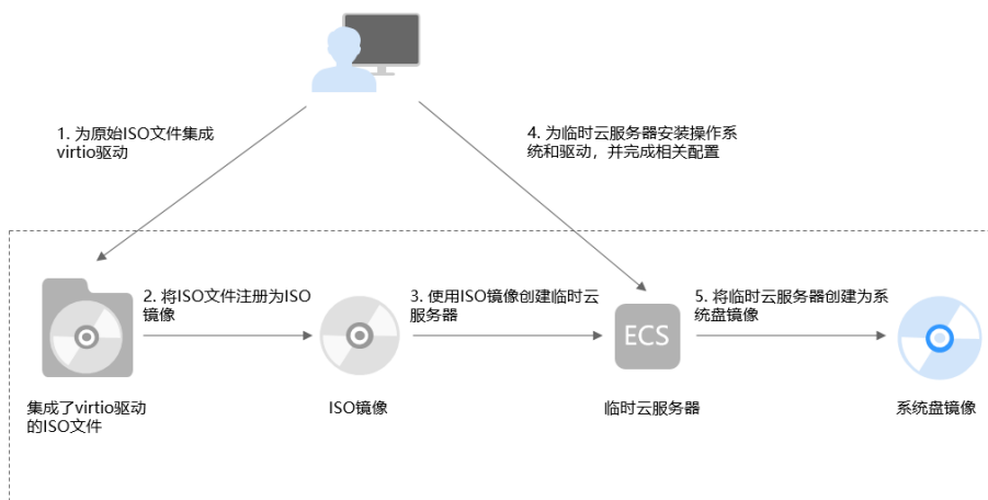
图 3-14 创建过程（Windows 系统盘镜像）
