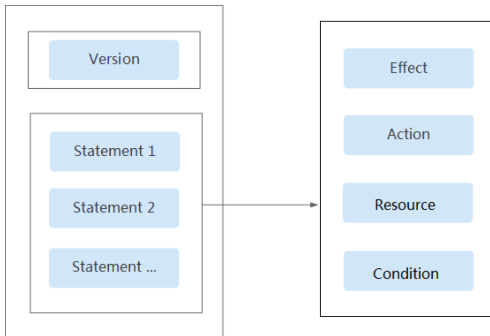
图3-6 策略结构
