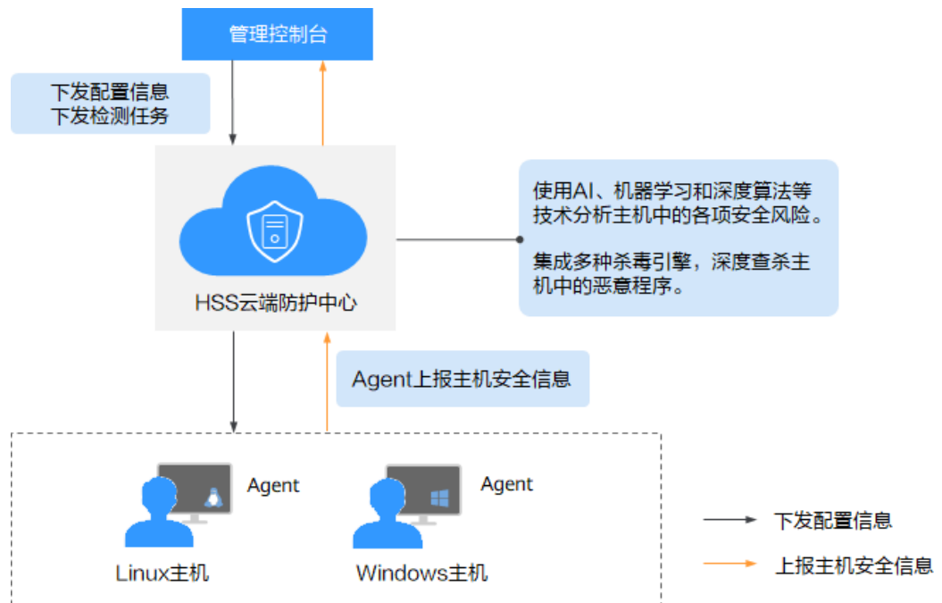
图 1-1 工作原理
