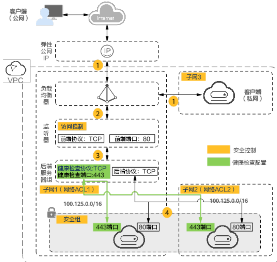
图 14-1 客户端通过负载均衡访问后端服务器示意图
