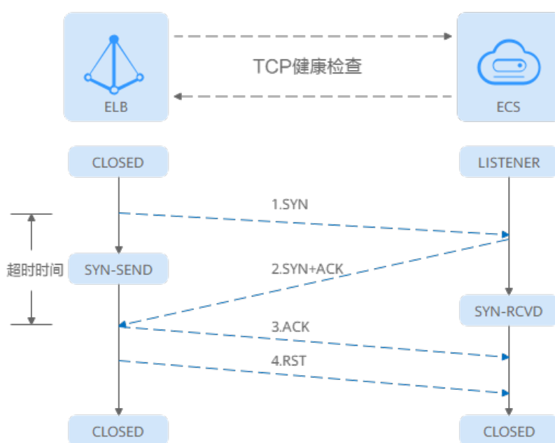
图 6-1 TCP 健康检查
