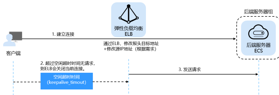
图 4-2 四层监听器超时时间示意图
