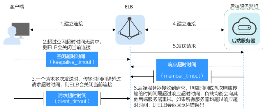
图 4-1 七层监听器超时时间示意图
