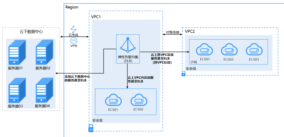
图 7-1 ELB 支持添加云上、云下的服务器
