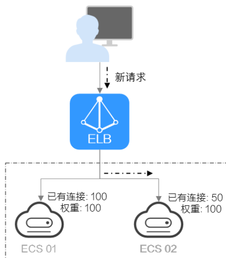
图 6-7 加权最少连接算法流量分发
