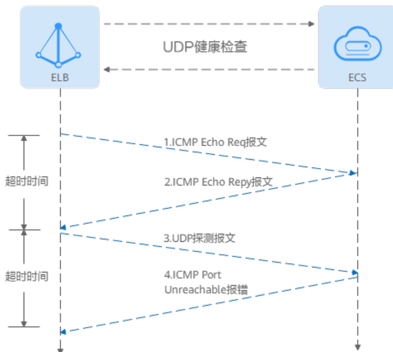
图 6-2 UDP 健康检查
