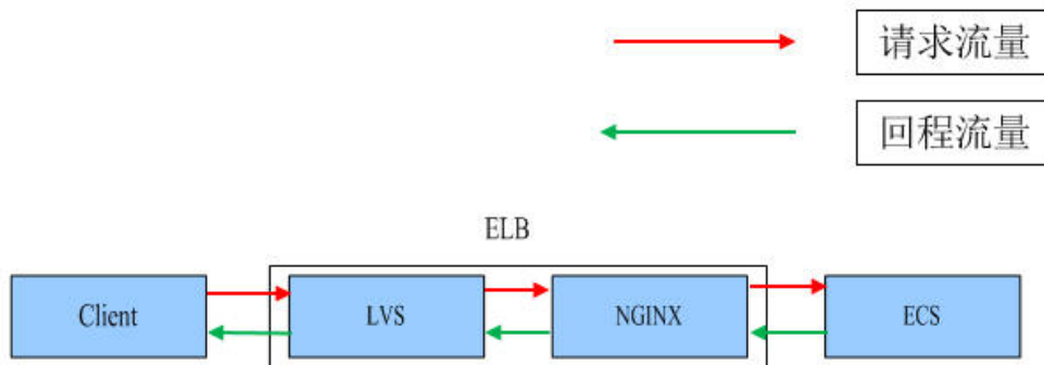
图 14-4 七层转发协议
