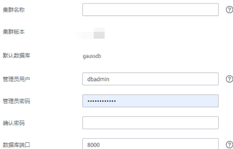
图 2-2 集群配置
