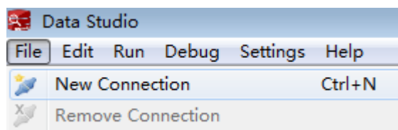
图 6-3 新建连接
