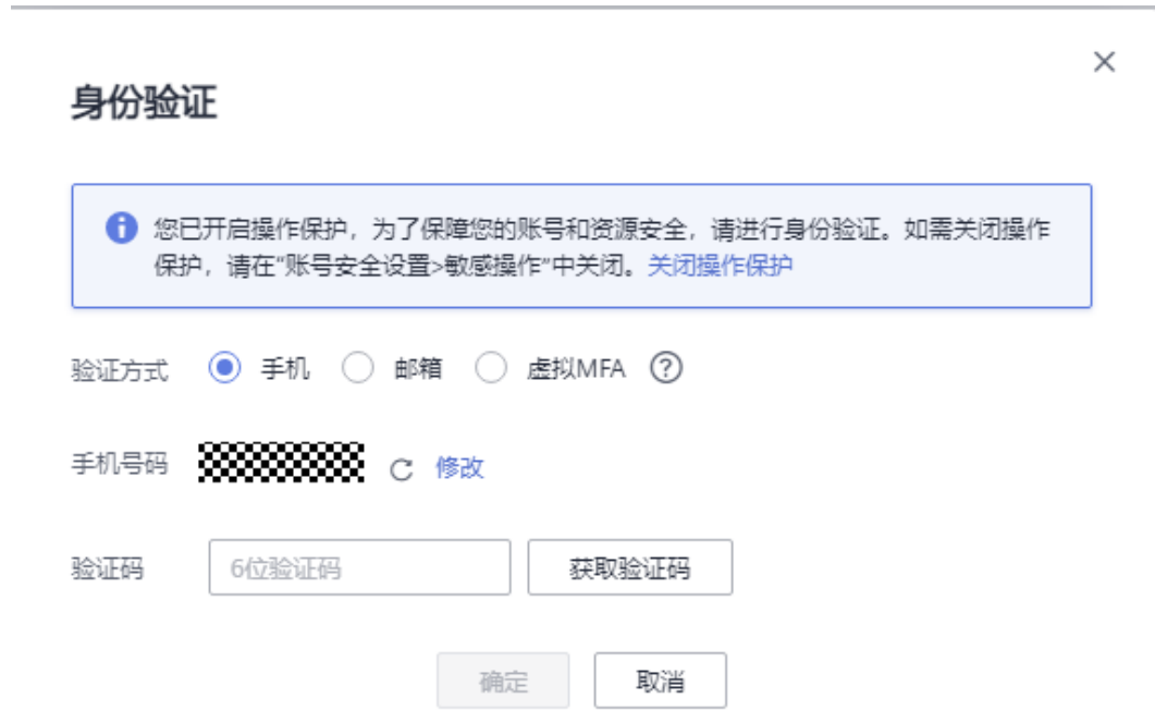
图 10-8 身份验证
