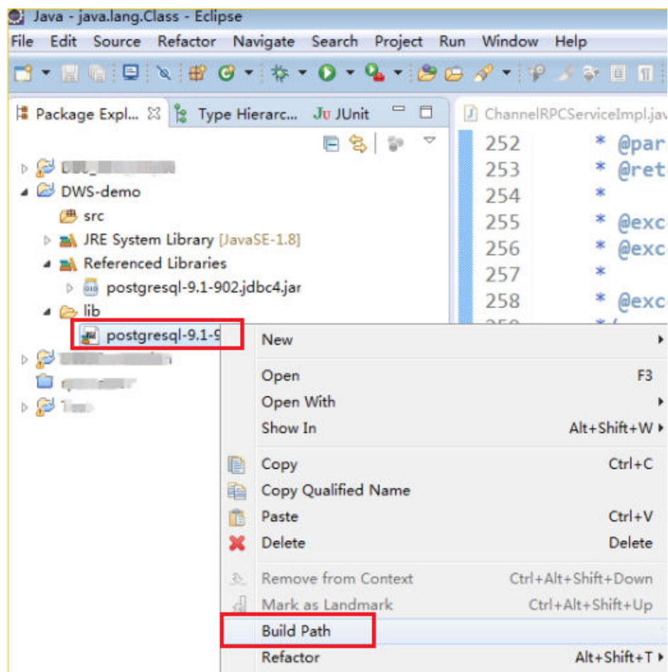
图 6-7 引用 jar 包
