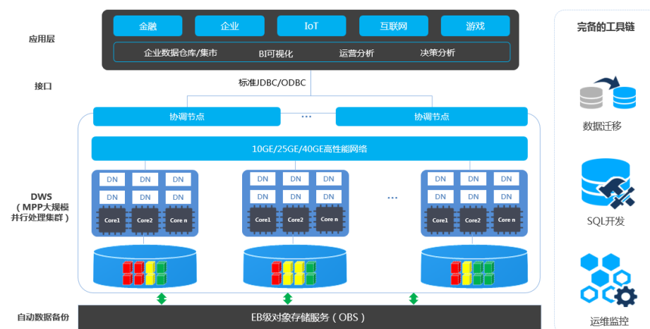
图 1-1 产品架构
