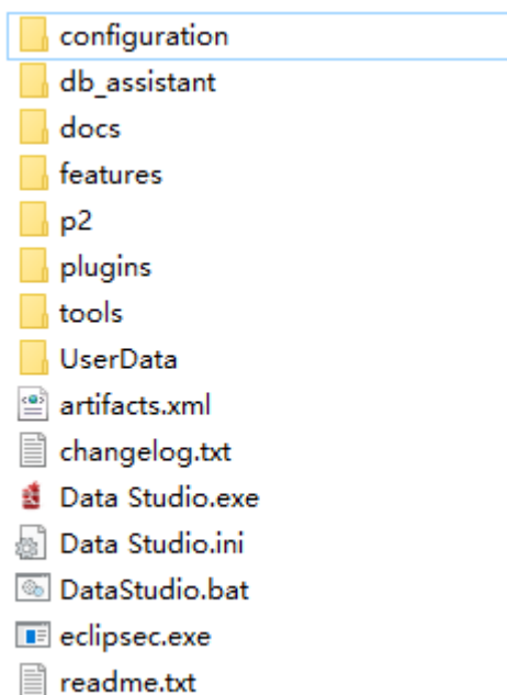
图 2-4 启动客户端
