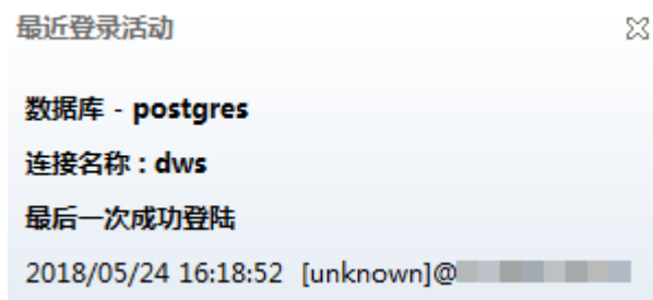
图 6-6 登录成功
