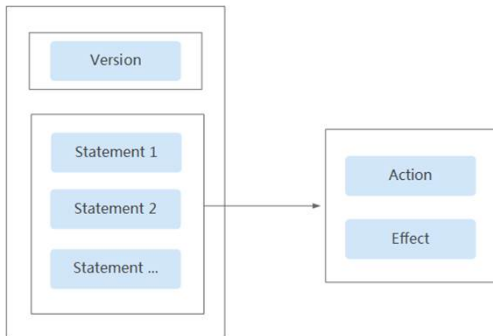
图 10-1 策略结构
