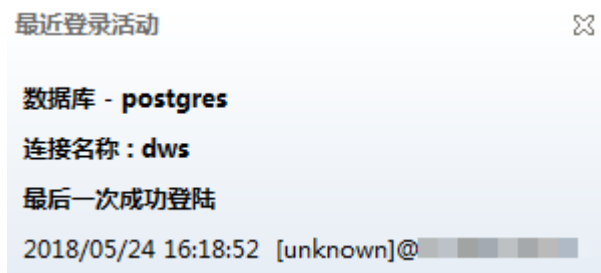
图 2-8 登录成功
