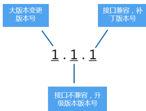
图 7-1 版本说明
