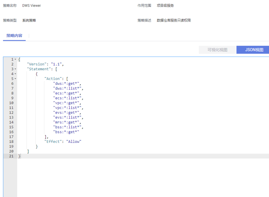
图 10-2 设置策略
