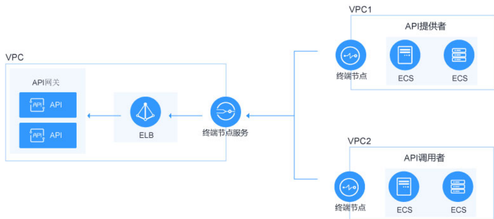
图 9-1 同一区域跨 VPC 访问
