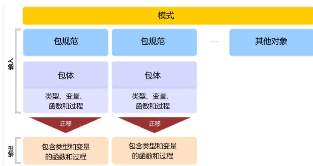
图 6-55 PL/SQL 包迁移
