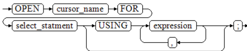
图 13-30 open_dynamic_cursor::=
