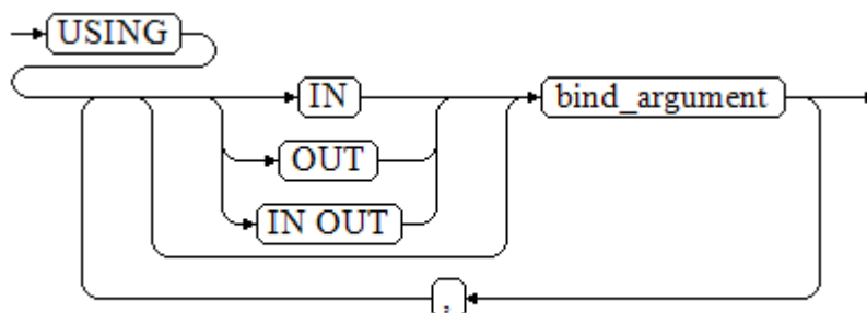
图 13-12 using_clause-3
