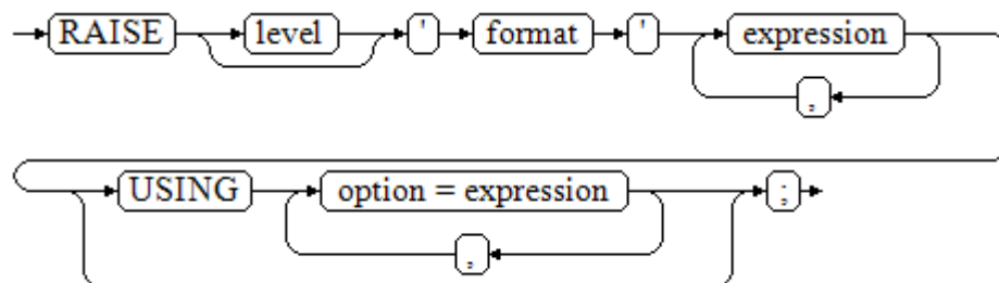
图 13-34 raise_format::=
