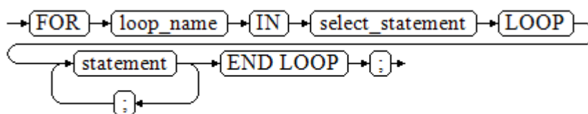
图 13-33 FOR_AS_loop::=
