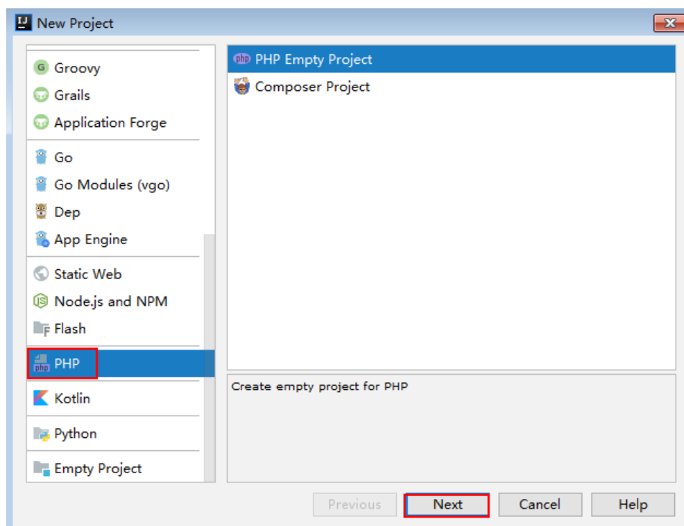
图 2-30 PHP
