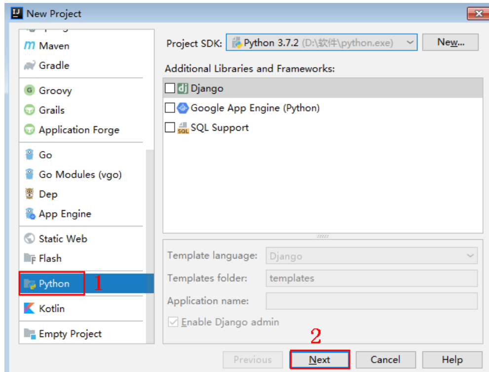
图 2-18 Python
