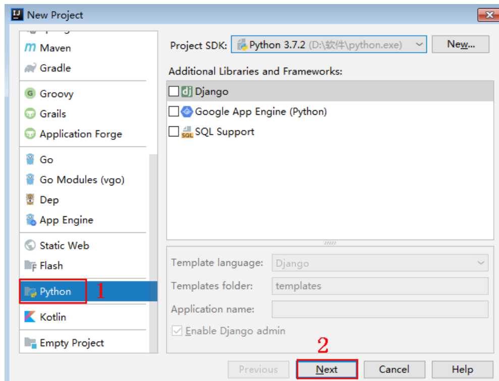
图 6-5 New Python
