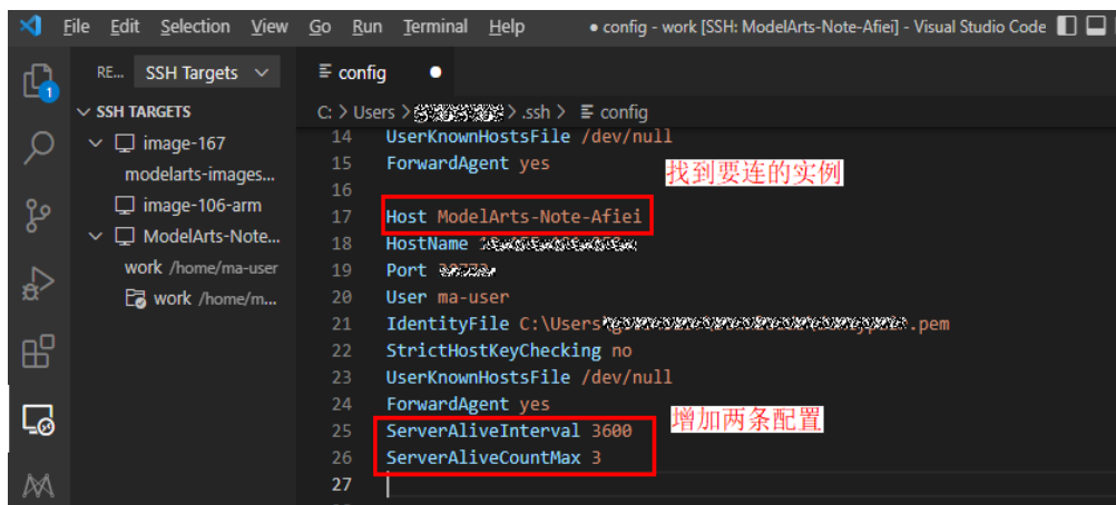
图 5-16 增加配置信息
