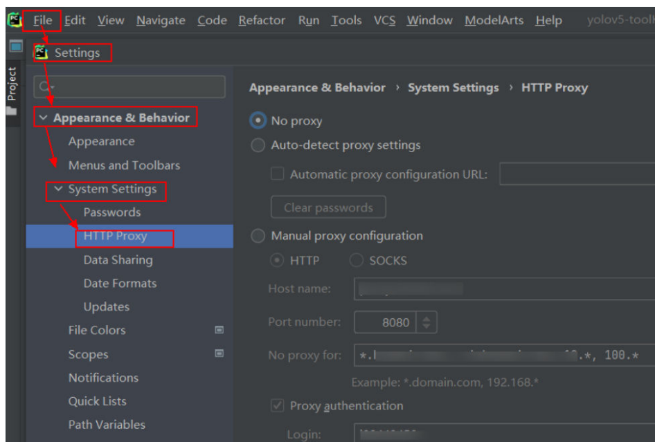
图 10-3 PyCharm 网络代理设置
