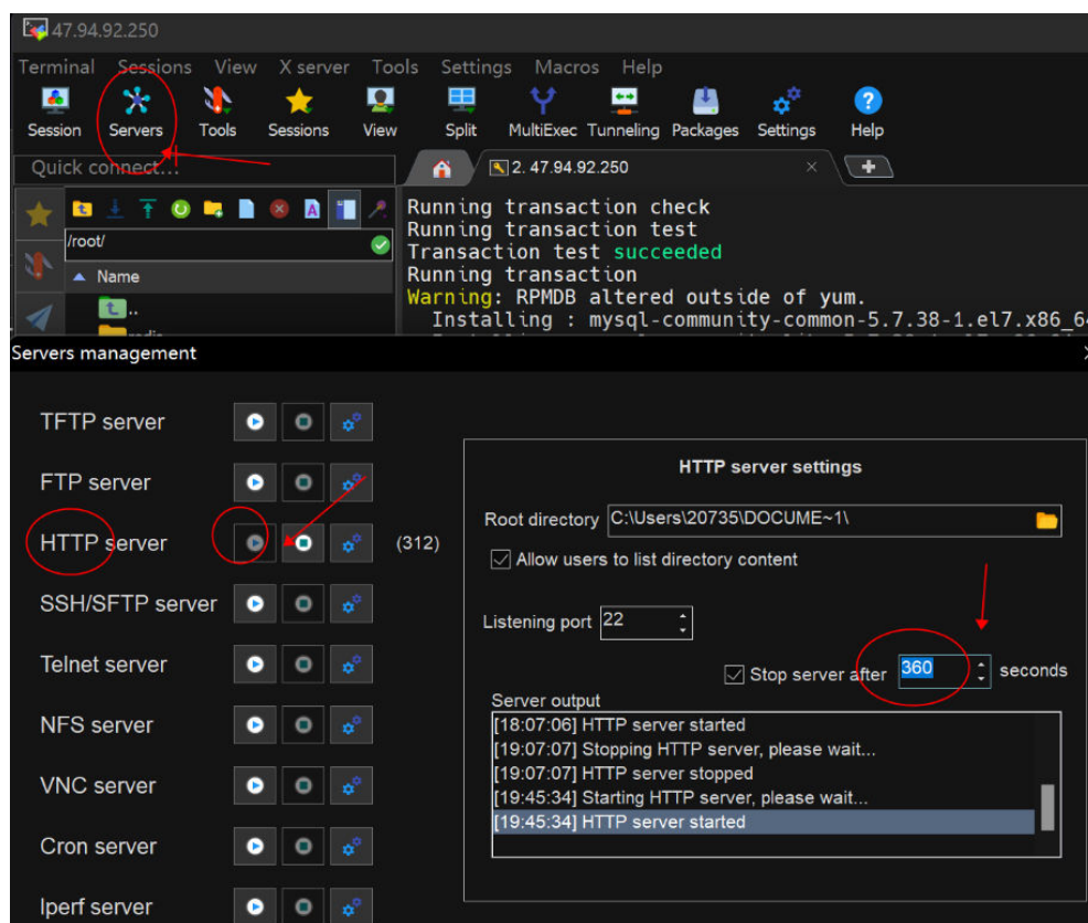
图 5-21 设置“Stop server after”
