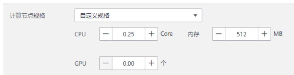
图 7-4 自定义规格
