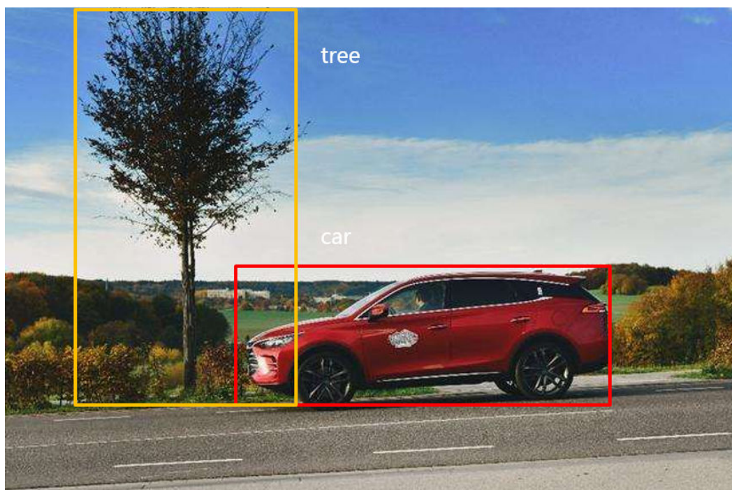
图 3-2 物体检测
