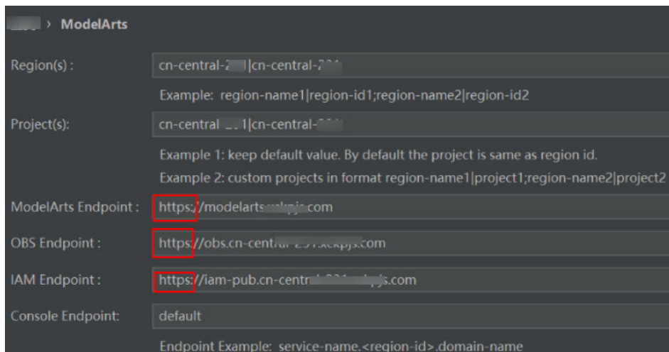
图 10-2 配置 ToolKit
