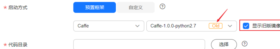
图 6-3 创建算法
