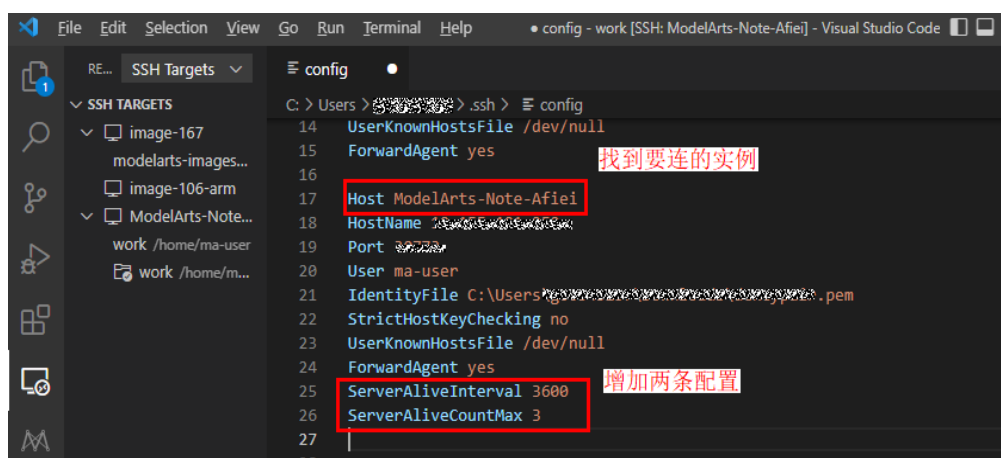
图 5-28 增加配置信息
