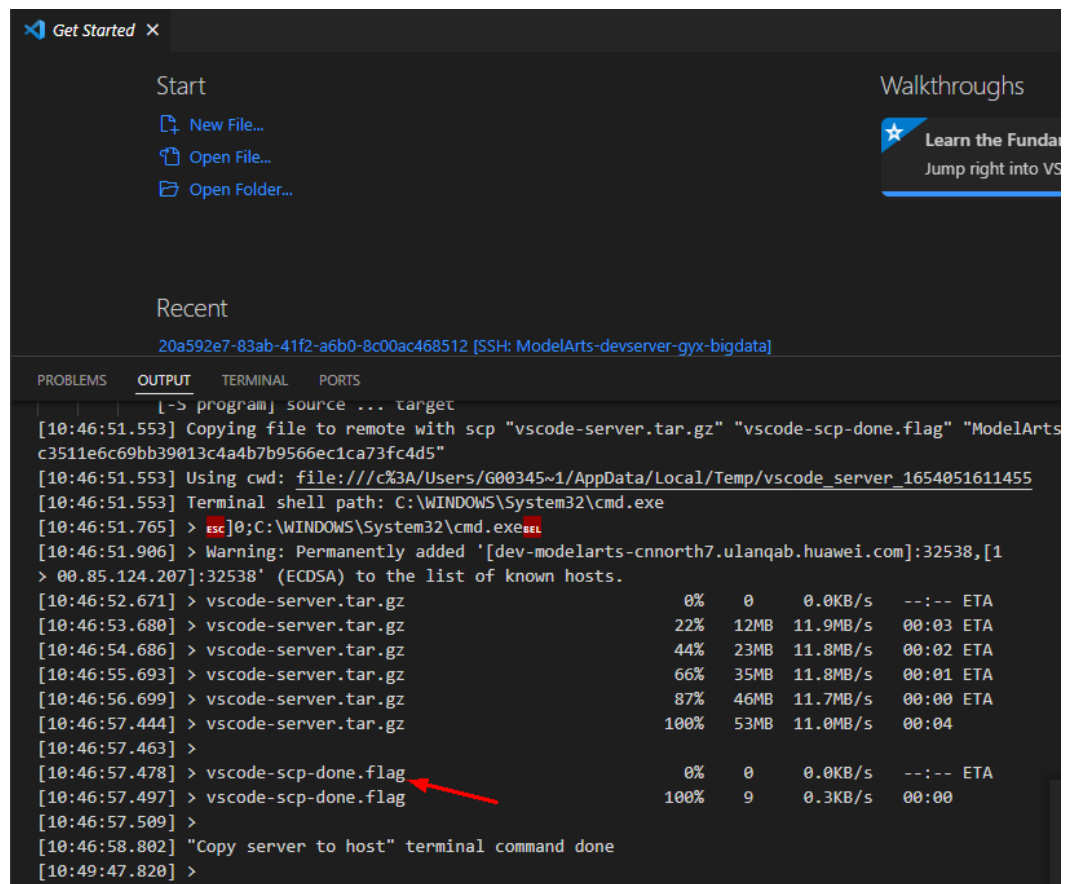
图 5-21 vscode-scp-done.flag 本地成功上传
