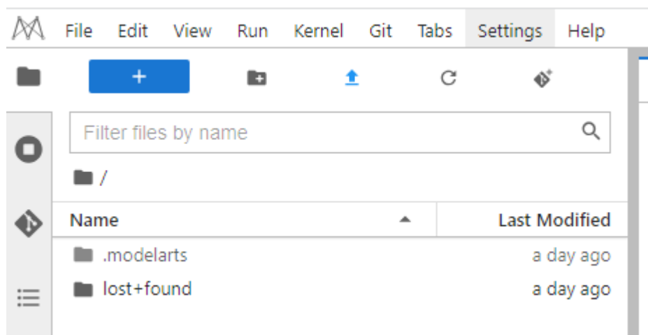
图 5-5 Notebook 的 JupyterLab
