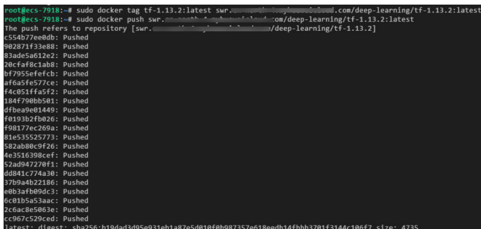
图 8-2 上传镜像
