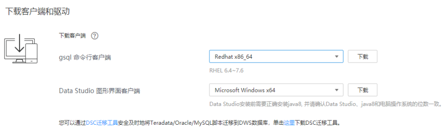
图 3-1 下载工具
