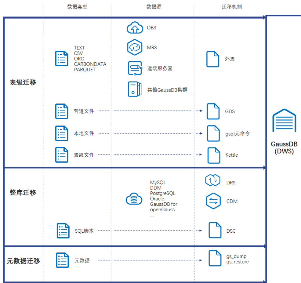
图 1-1 数据迁移示意图
