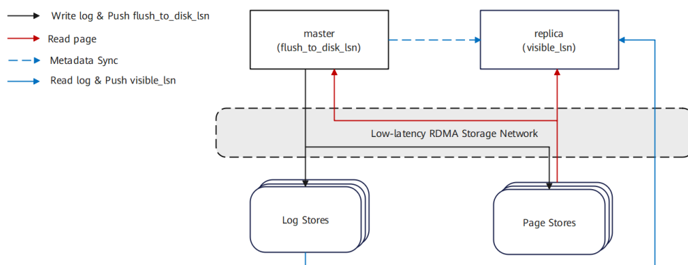
图 2-25 只读落后自愈技术原理图
