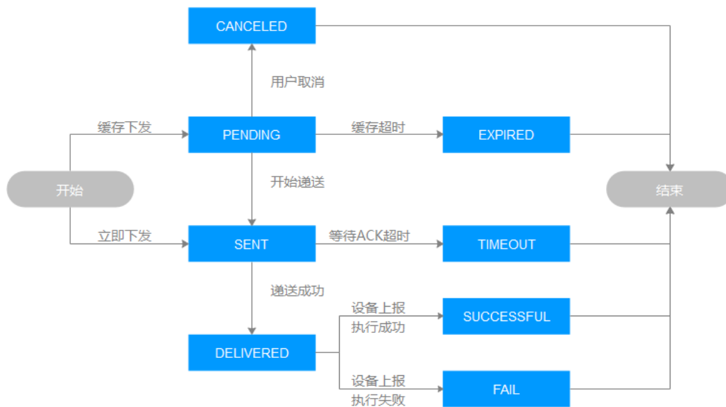
图 8-6 命令状态转换图
