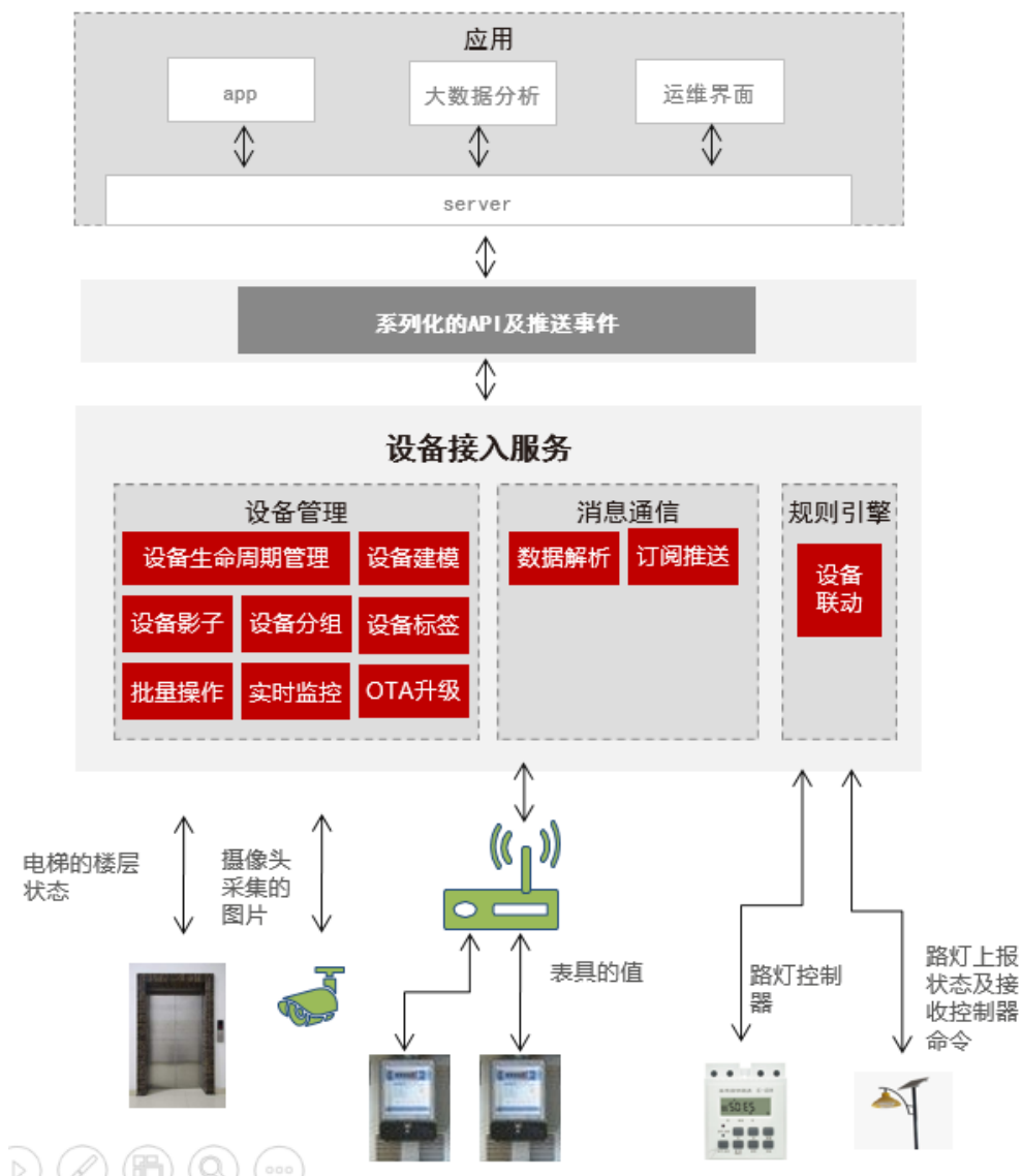
图 2-1 设备 + IoT 平台 + 应用
