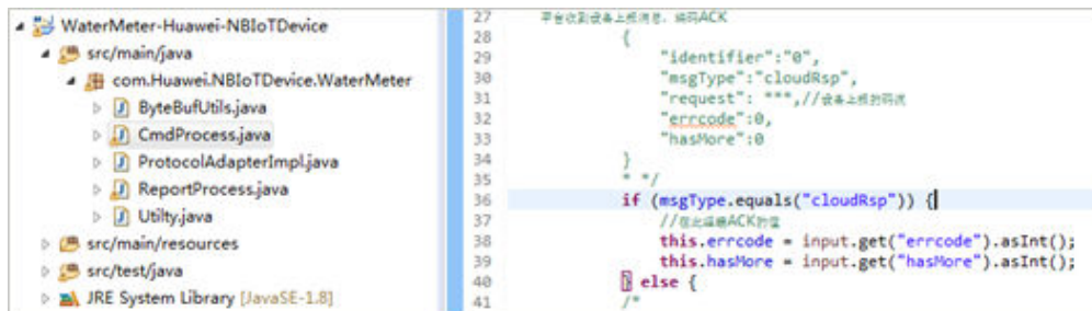
图 8-3 插件代码样例
