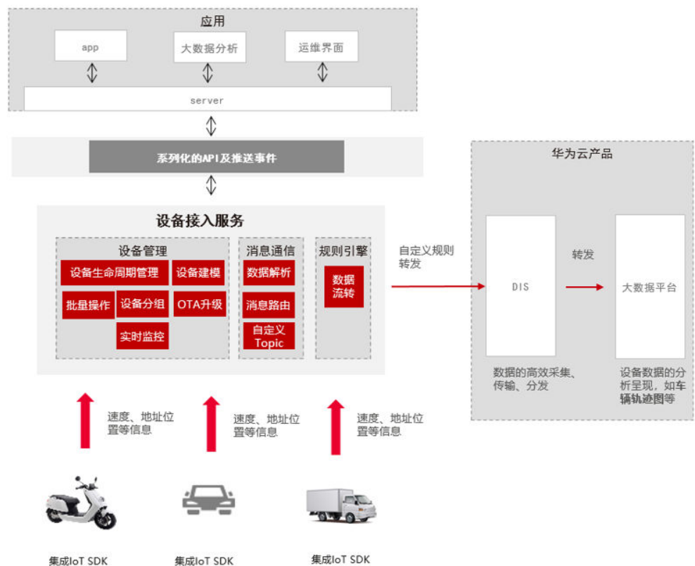
图 2-3 设备 + IoT 平台 + 第三方云服务 + 应用
