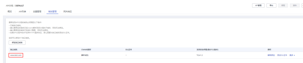
图 3-4 域名示例
