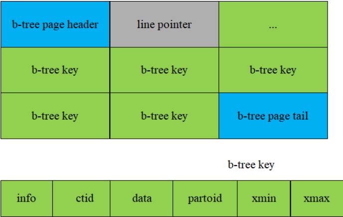
图 6-1 RCR UBTree 多版本管理
