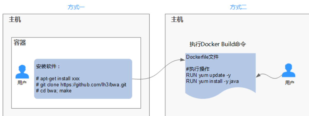
图 7-3 使用 Dockerfile 方式构建
