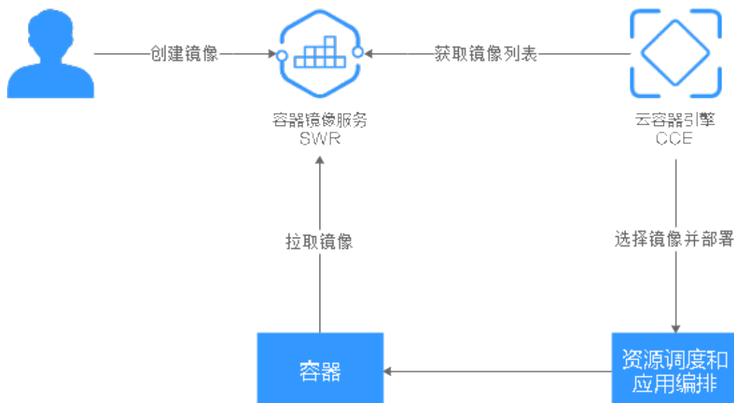
图 1-2 SWR 与 CCE 配合使用示意图
