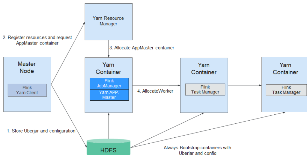
图 1-16 Flink 基于 YARN 的集群部署
