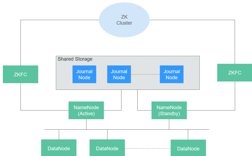
图 1-40 HA HDFS 结构
