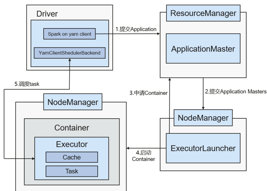
图 1-119 Spark on yarn-client 运行框架
