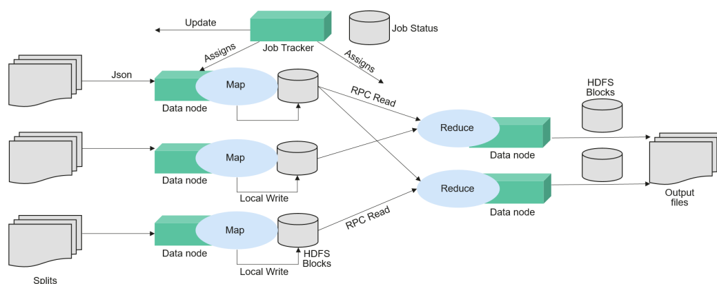
图 1-74 分布式批处理引擎
