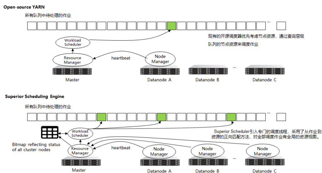
图 1-134 Superior Scheduler 性能对比
