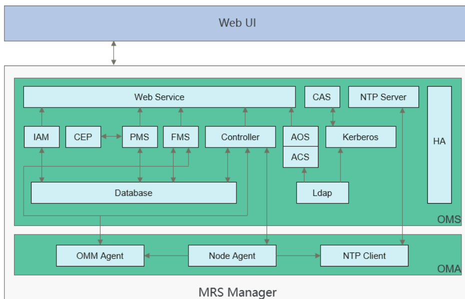
图 1-73 Manager 逻辑架构
