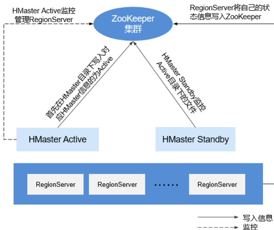
图 1-141 ZooKeeper 和 HBase 的关系
