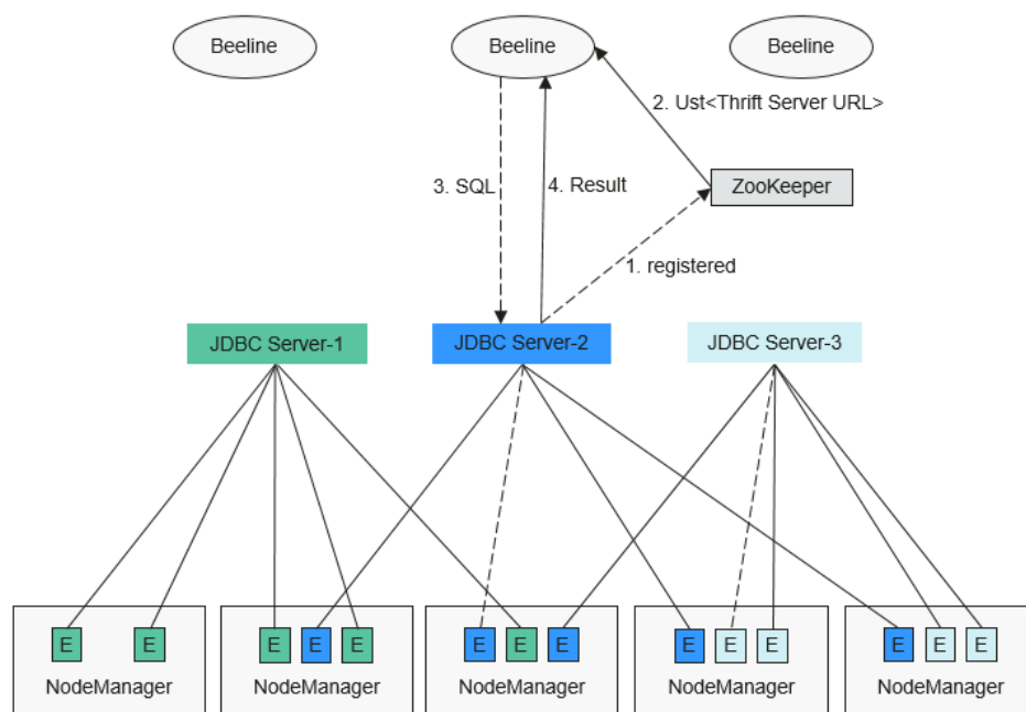
图 1-96 Spark JDBCServer HA
