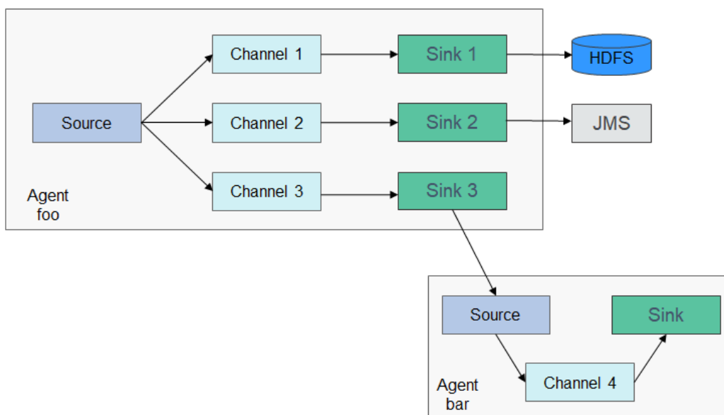
图 1-26 Flume 结构图
