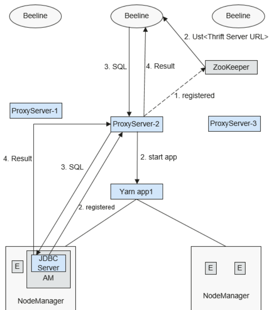
图 1-115 Spark JDBCServer 多租户
