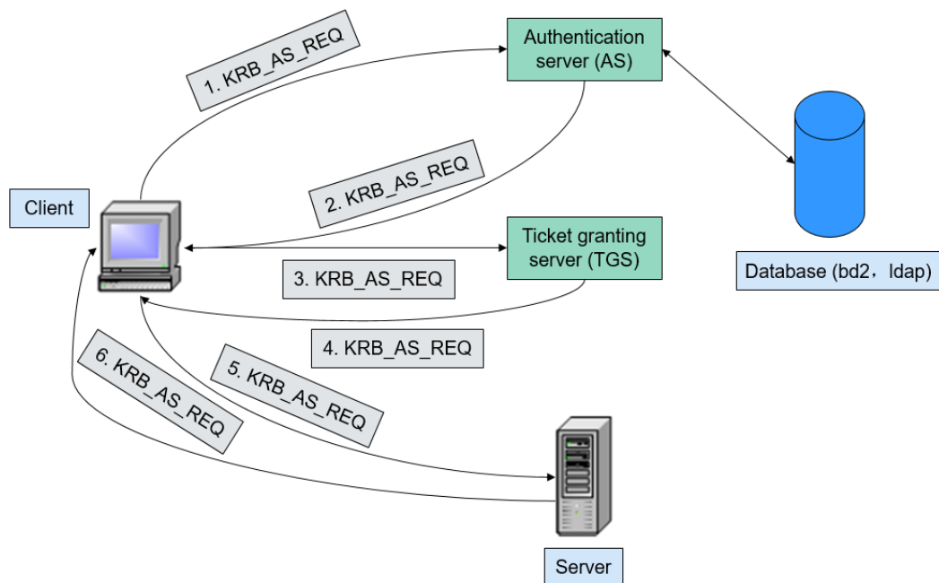
图 1-68 认证流程图
