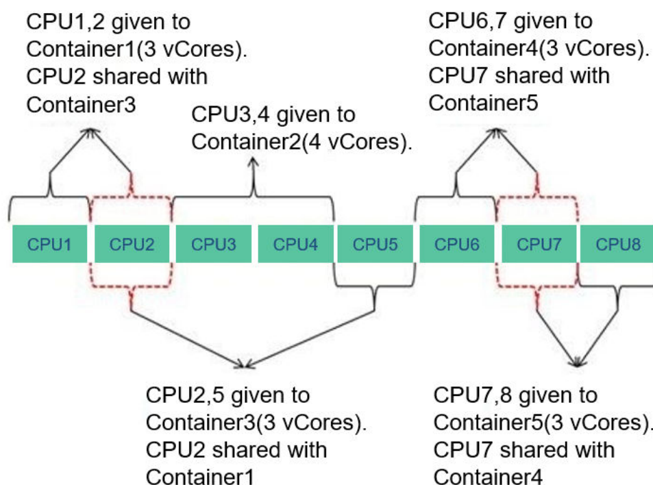
图 1-136 CPU 配额
