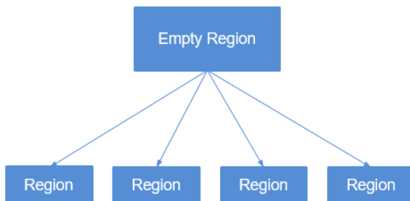
图 1-37 多点分割
