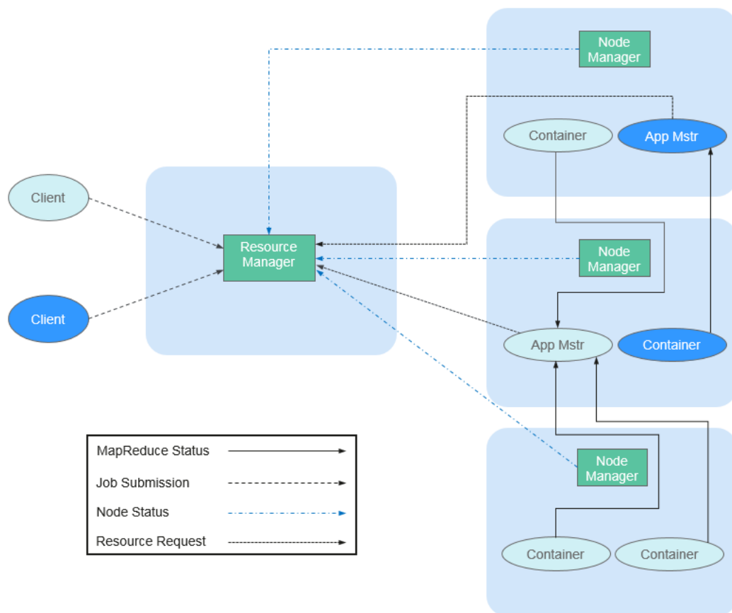
图 1-127 YARN 结构
