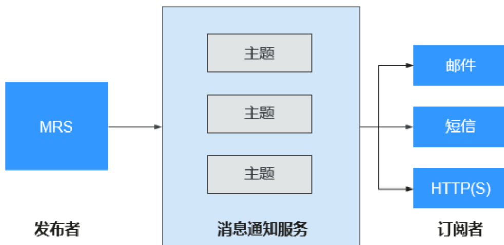
图 1-143 实现过程
