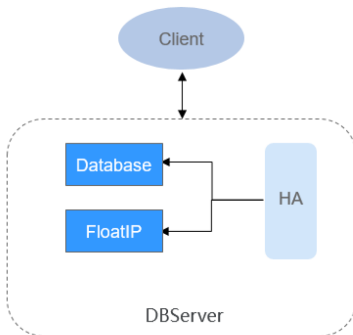
图 1-9 DBService 结构
