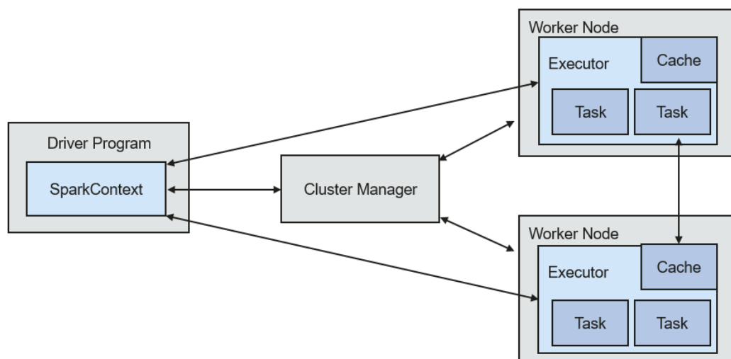
图 1-102 Spark 架构
