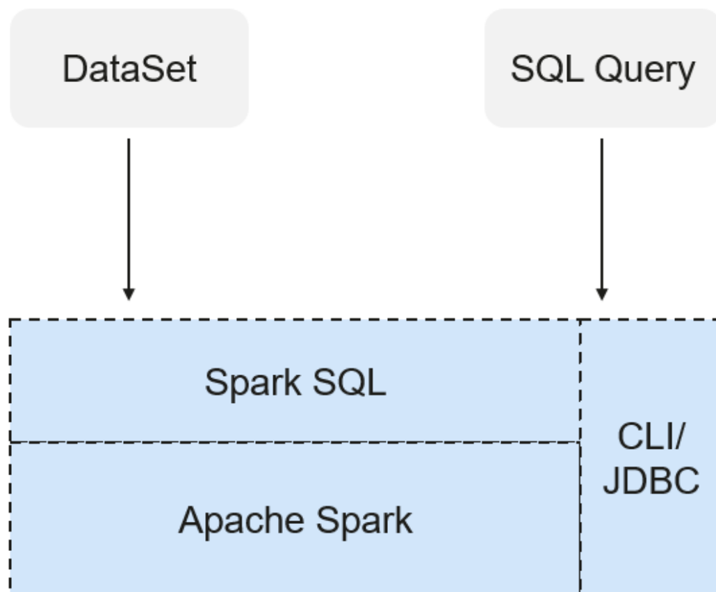
图 1-108 SparkSQL 和 DataSet
