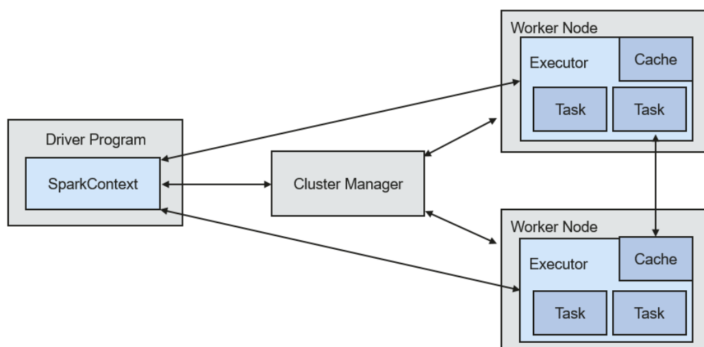
图 1-84 Spark 结构
