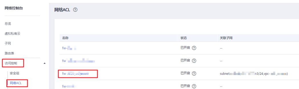
图 4-2 网络 ACL
