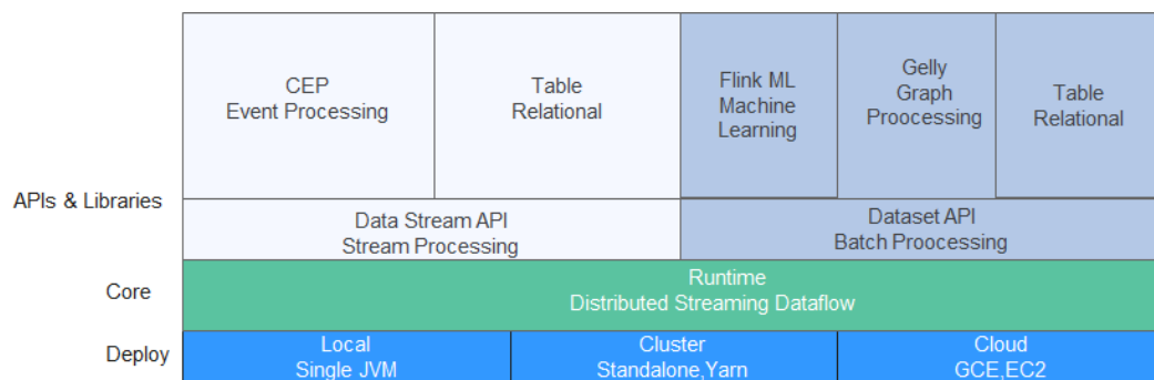
图 1-10 Flink 技术栈
