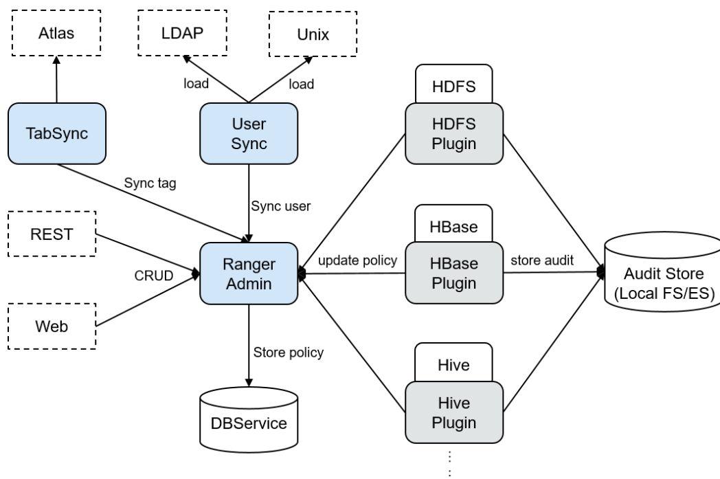
图 1-82 Ranger 结构
