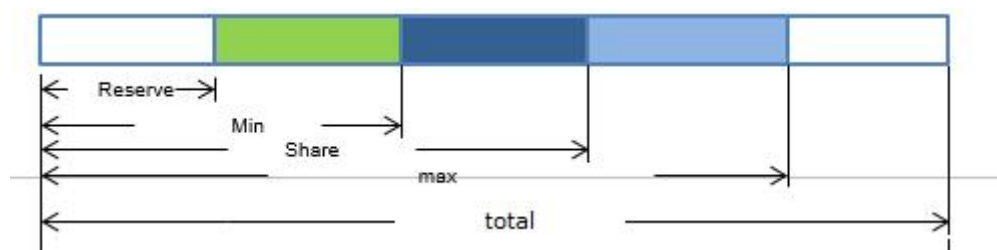
图 1-135 策略示意图
