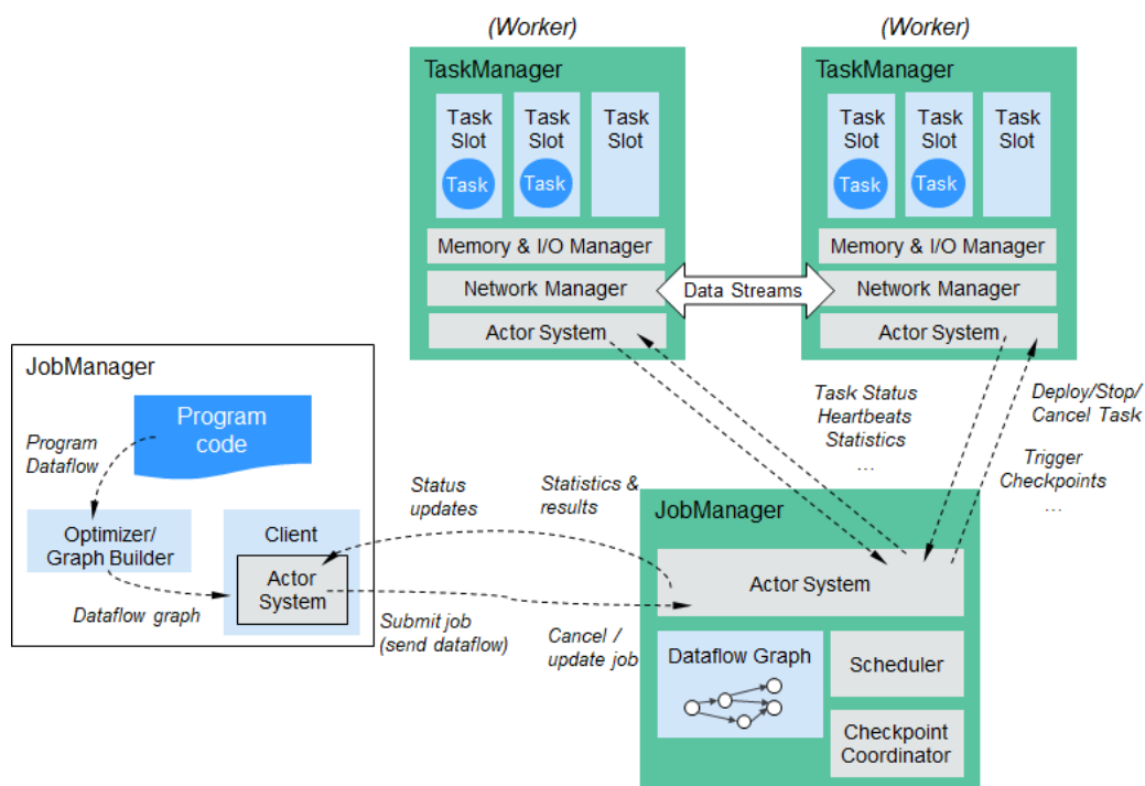
图 1-11 Flink 结构
