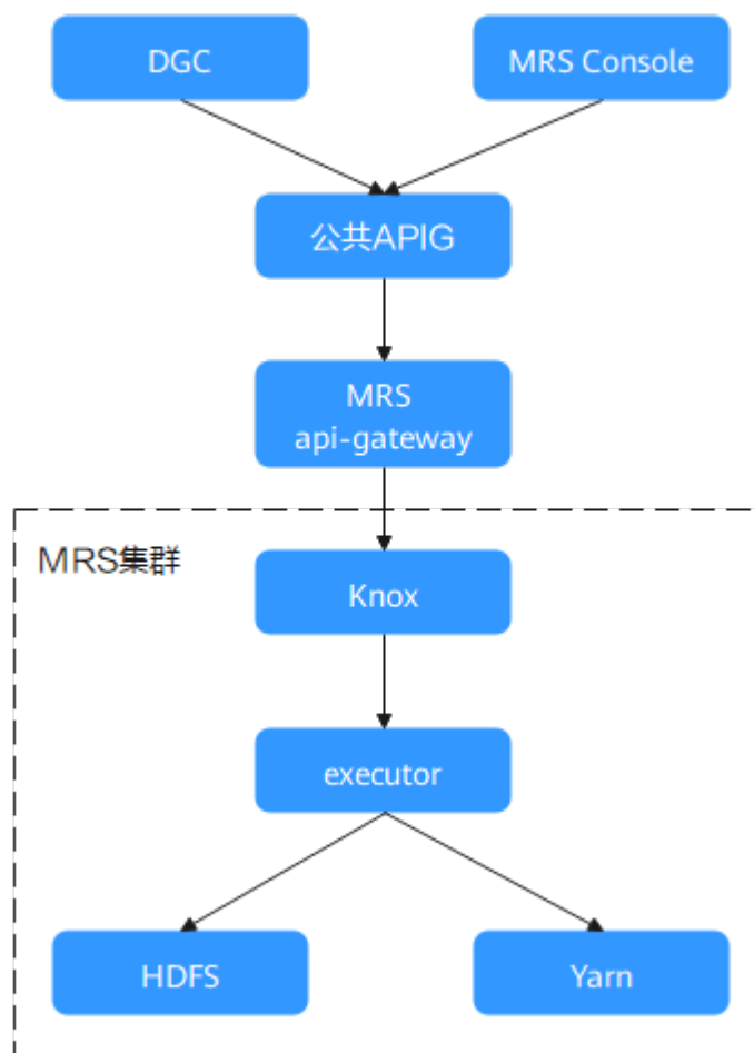
图 15-7 作业流程
