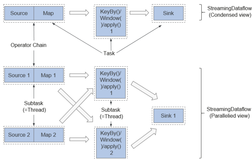
图 1-14 Operator chain
