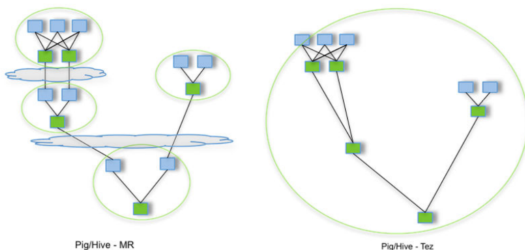
图 1-126 Hive 基于 MapReduce 提交任务和基于 Tez 提交任务流程图
