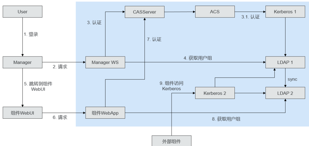
图 1-67 安全认证场景架构
