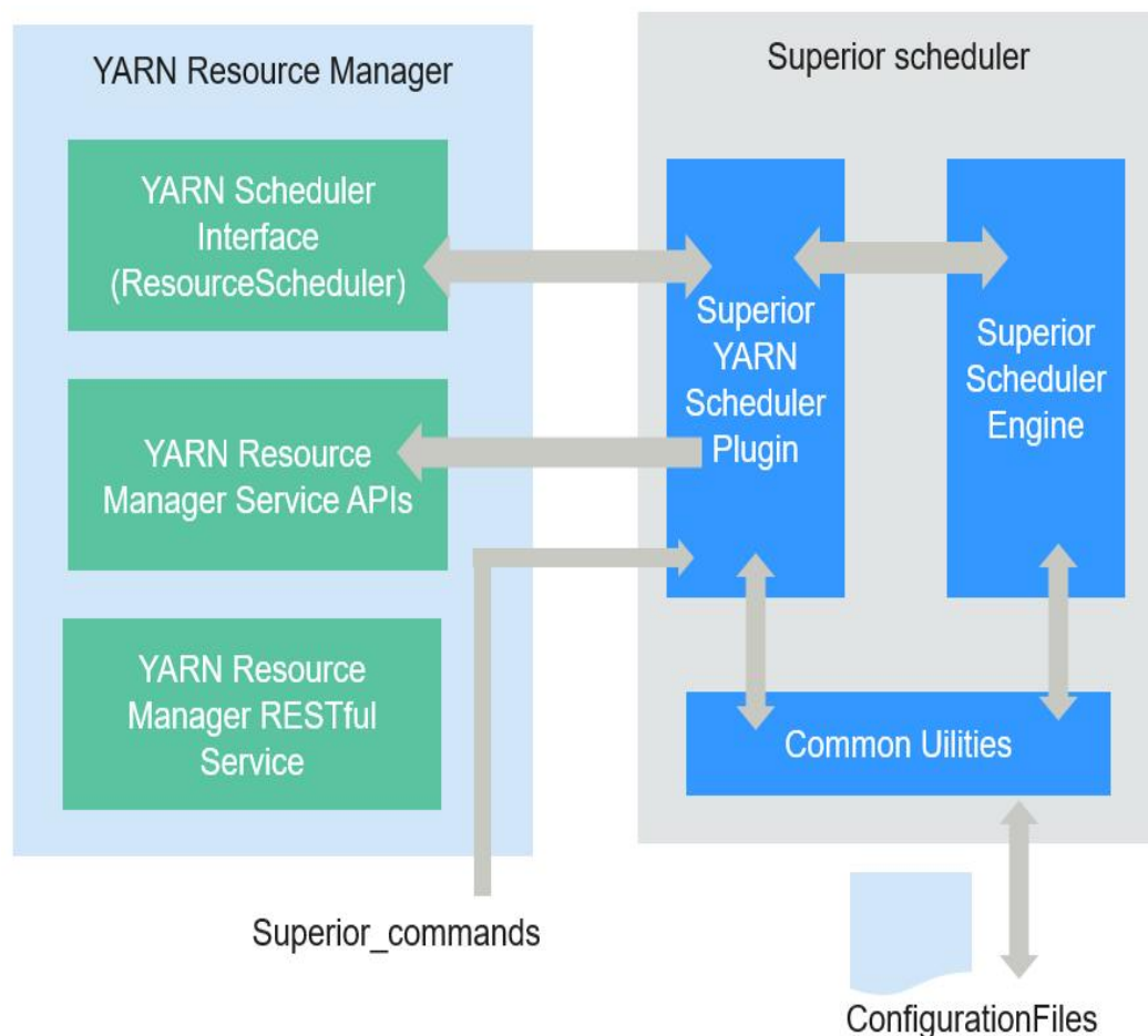
图 1-133 Superior Scheduler 内部架构
