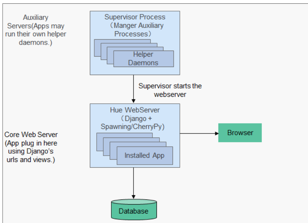
图 1-62 Hue 架构示意图
