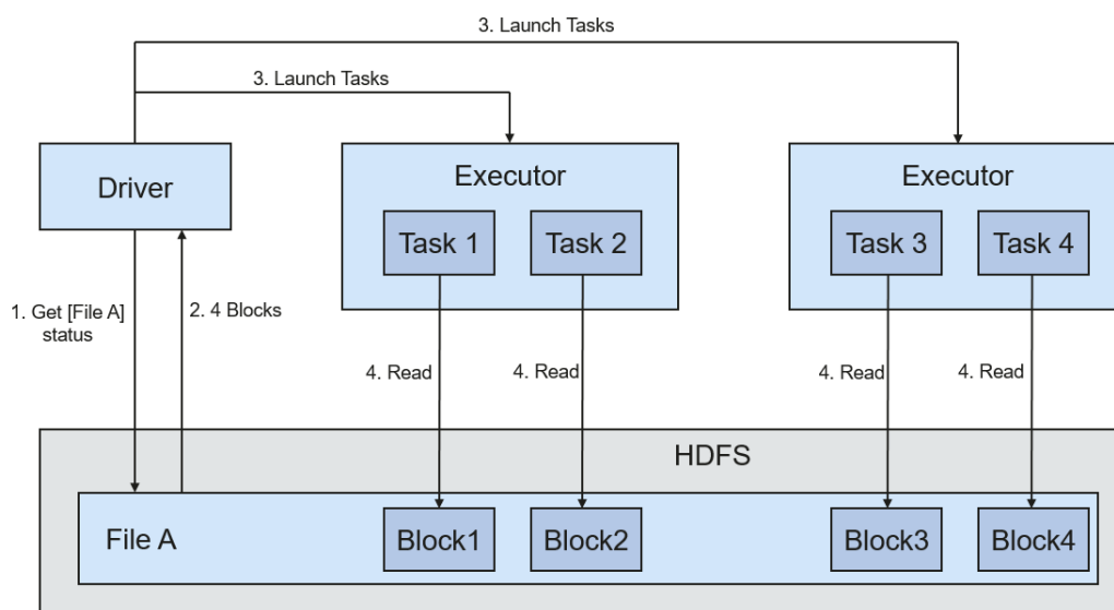
图 1-116 读取文件过程
