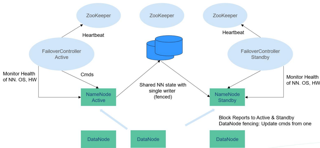
图 1-43 典型的 HA 部署方式
