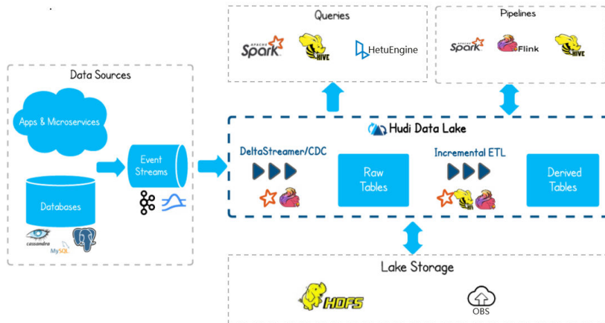
图 1-61 Hudi 基本架构
