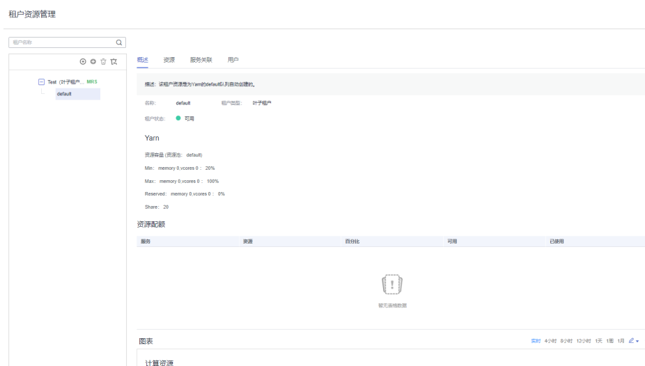
图 9-8 多租户管理
