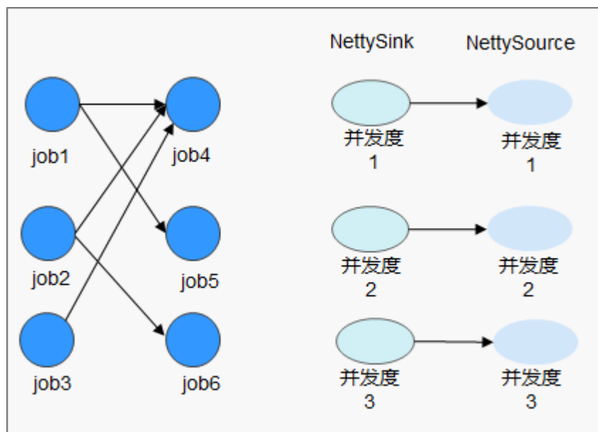
图 1-24 关系图
