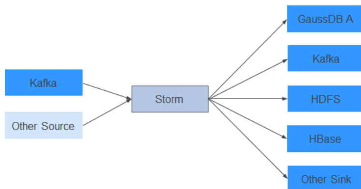
图 1-125 组件关系图
