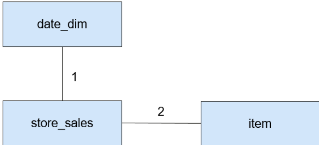
图 1-58 Join 关系
