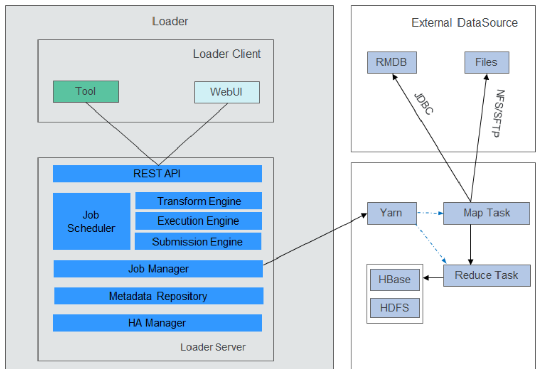
图 1-72 Loader 模型
