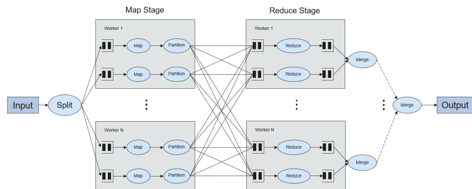
图 1-113 算法流程
