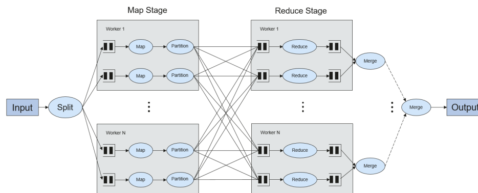
图 1-95 算法流程
