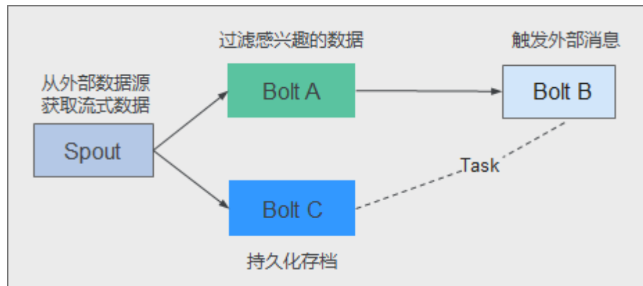
图 1-123 Topology
