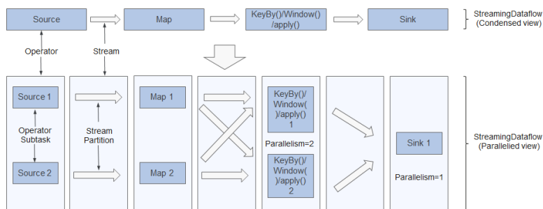
图 1-13 Operator
