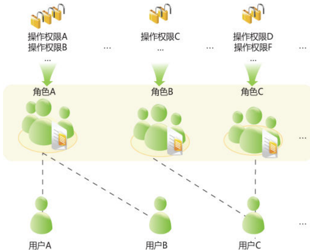
图 9-14 权限模型
