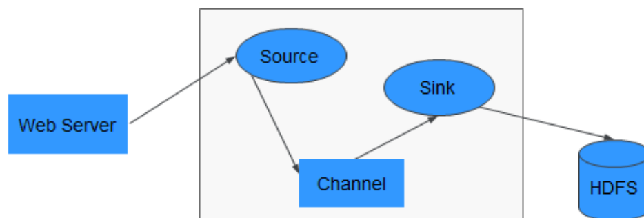
图 1-25 Flume-NG 架构
