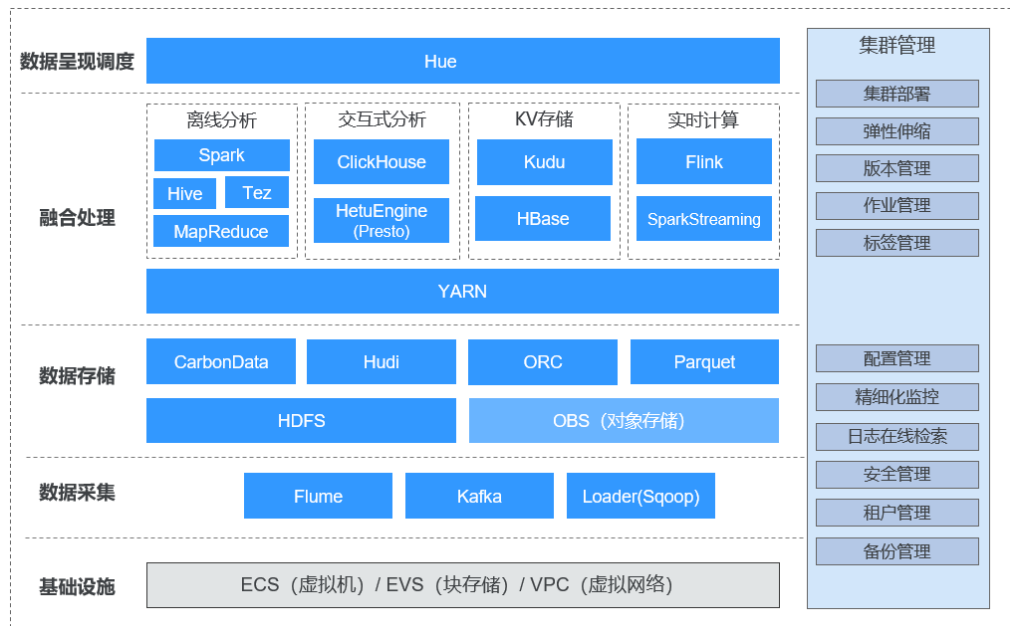
图 1-1 MRS 架构
