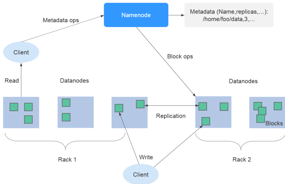
图 1-42 HDFS 架构
