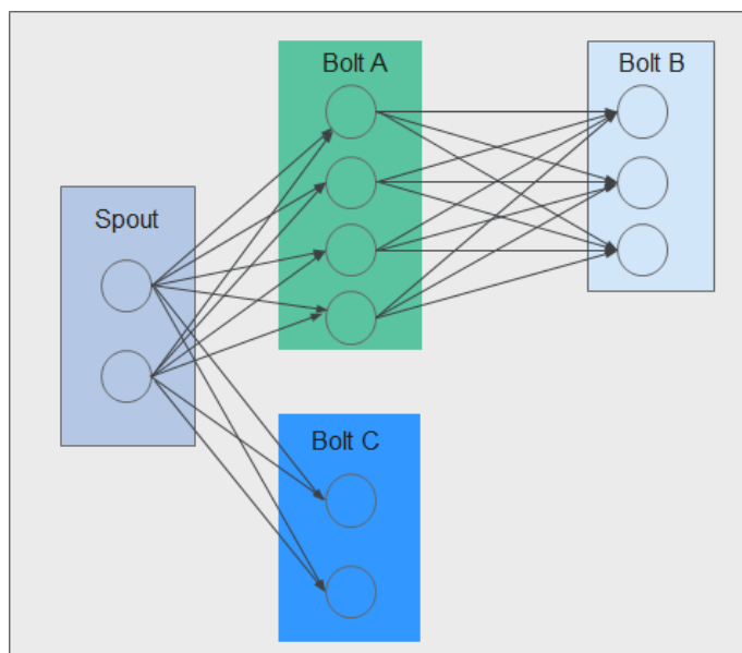
图 1-124 Topology 示意图
