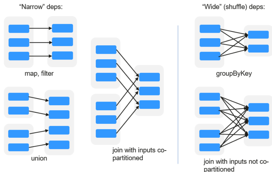
图 1-111 RDD 的依赖
