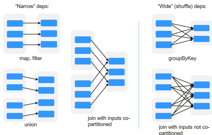
图 1-93 RDD 的依赖
