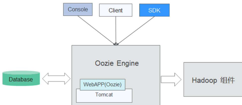
图 1-79 Oozie 框架
