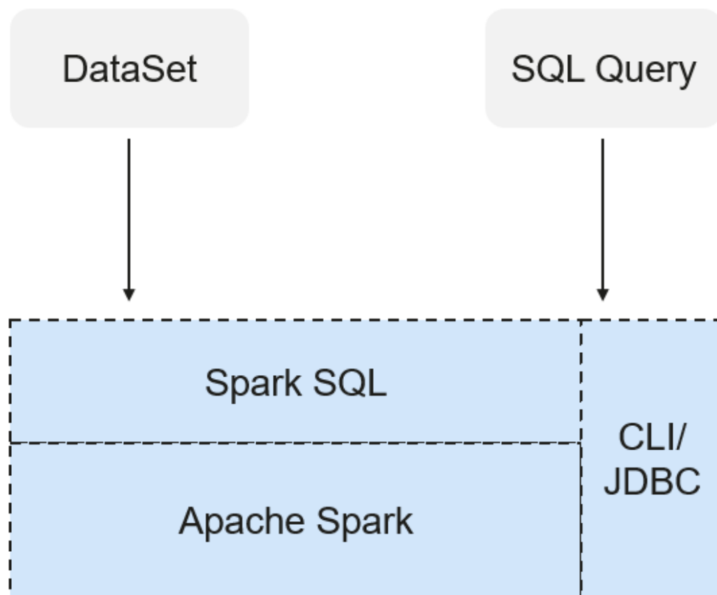
图 1-90 SparkSQL 和 DataSet
