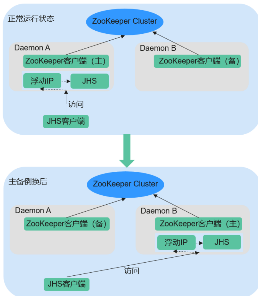
图 1-76 JobHistoryServer HA 主备倒换的状态转移过程
