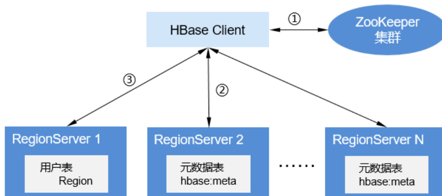
图 1-33 数据操作流程
