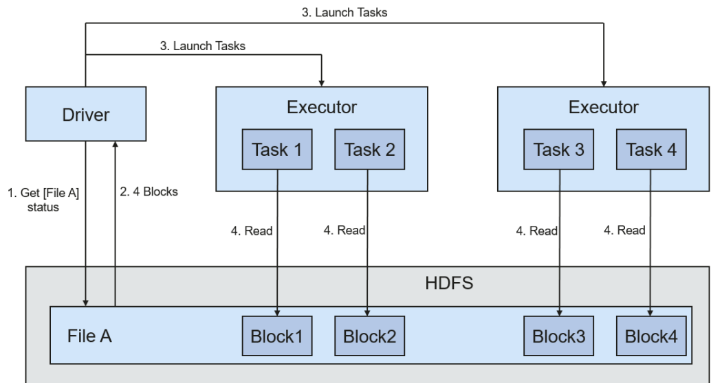
图 1-98 读取文件过程
