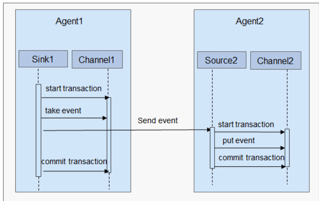
图 1-28 Agent 数据传输流程
