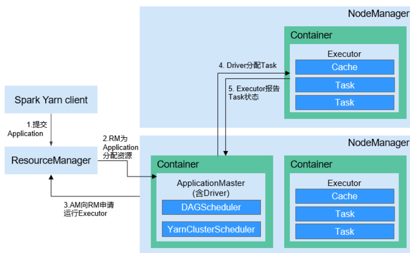
图 1-130 Spark on yarn-cluster 运行框架
