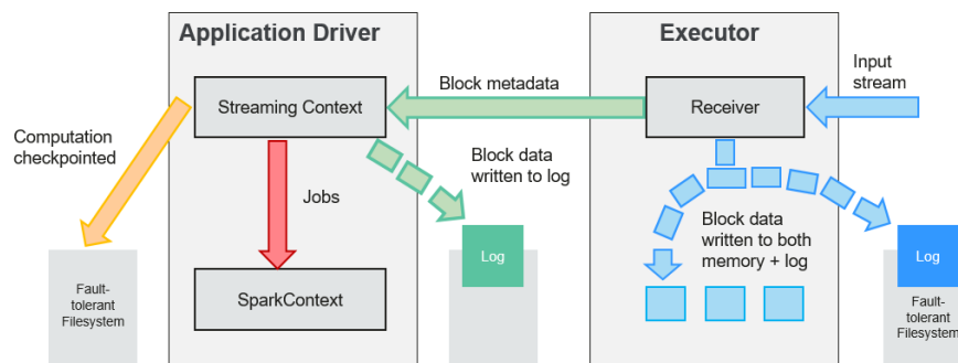
图 1-88 数据传输生命周期
