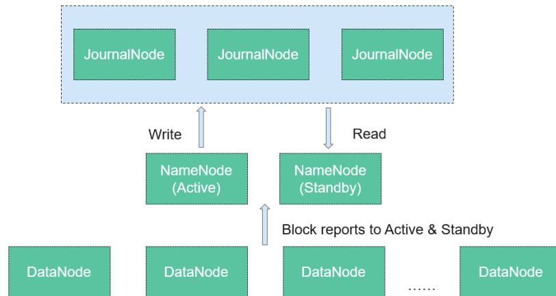
图 1-42 基于 QJM 的 HDFS 架构
