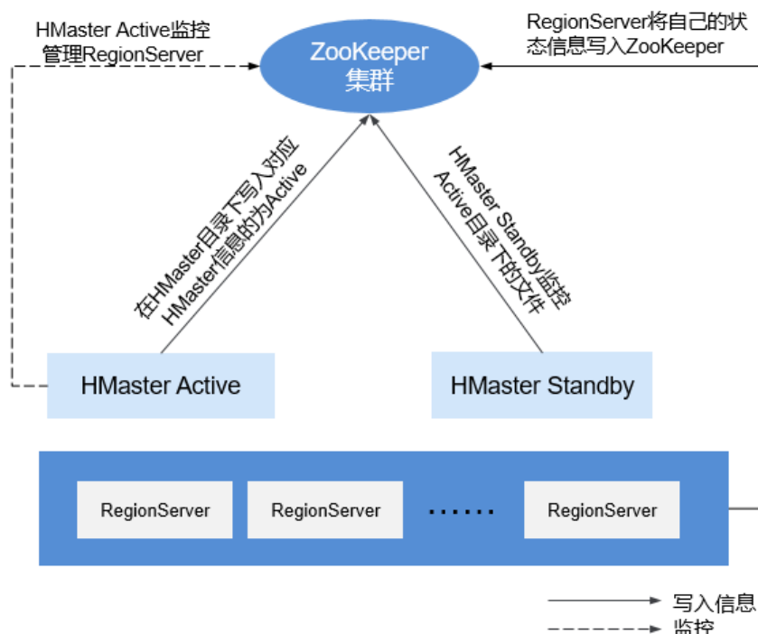
图 1-36 HBase 和 ZooKeeper 的关系
