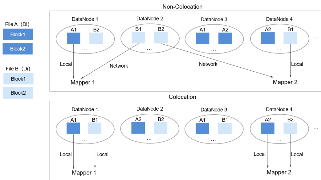
图 1-49 非同分布与同分布数据块分布对比
