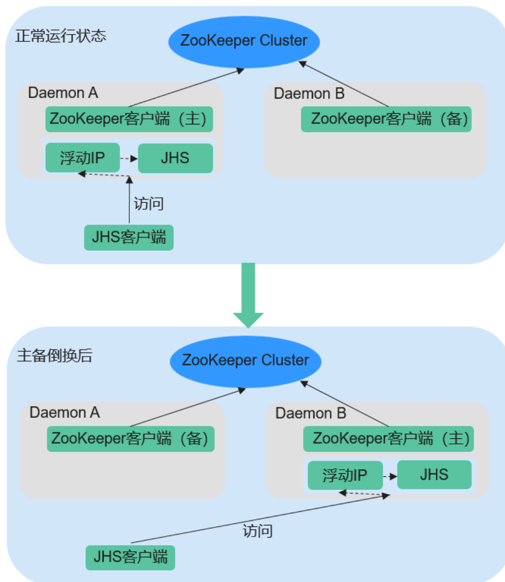
图 1-77 JobHistoryServer HA 主备倒换的状态转移过程
