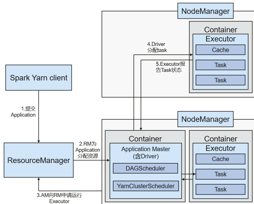
图 1-101 Spark on yarn-cluster 运行框架
