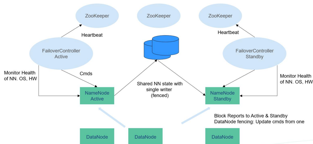
图 1-44 典型的 HA 部署方式
