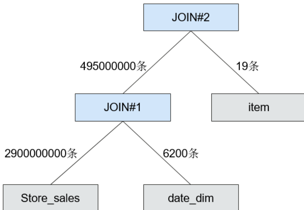
图 1-60 未开启 CBO
