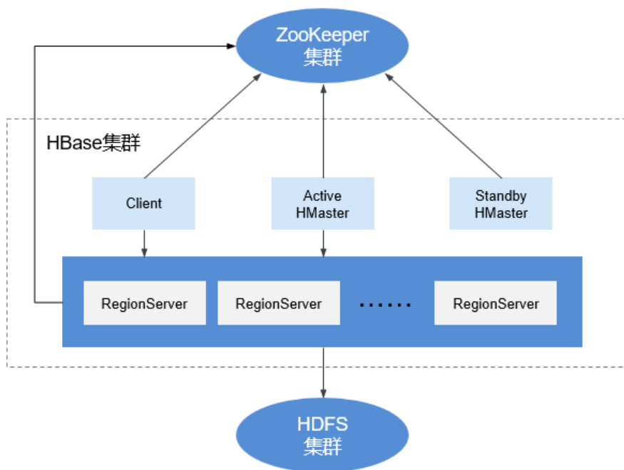
图 1-30 HBase 结构
