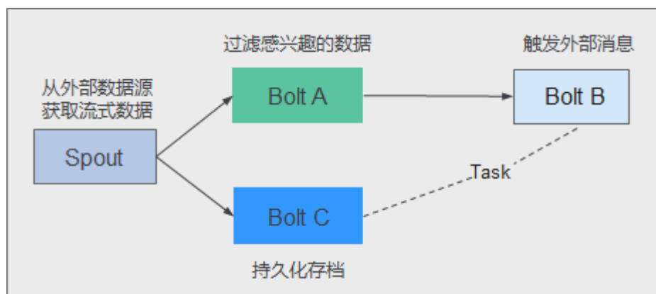
图 1-124 Topology
