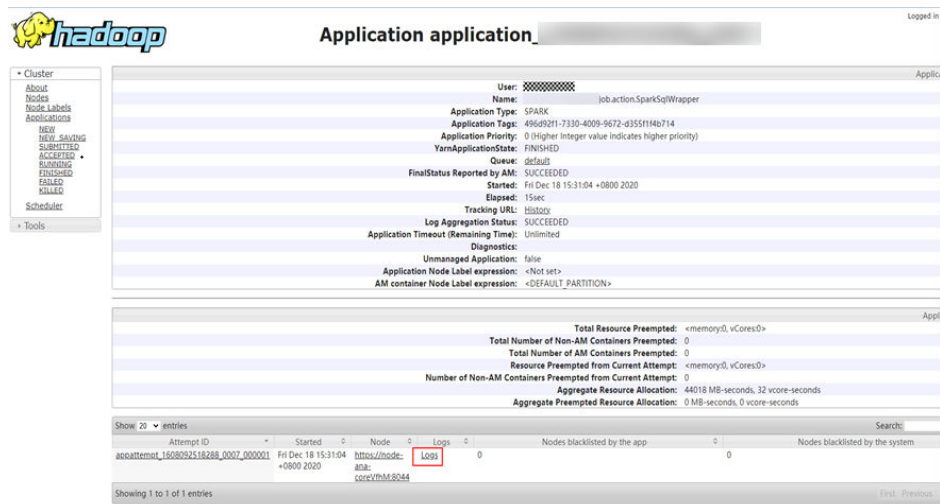
图 15-10 任务日志
