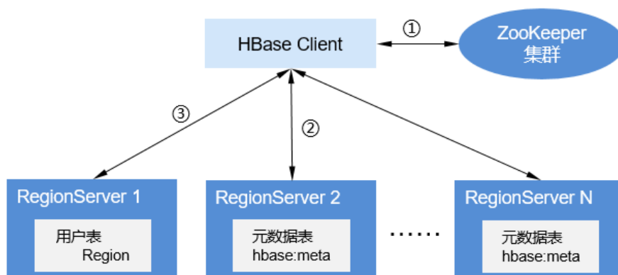
图 1-34 数据操作流程
