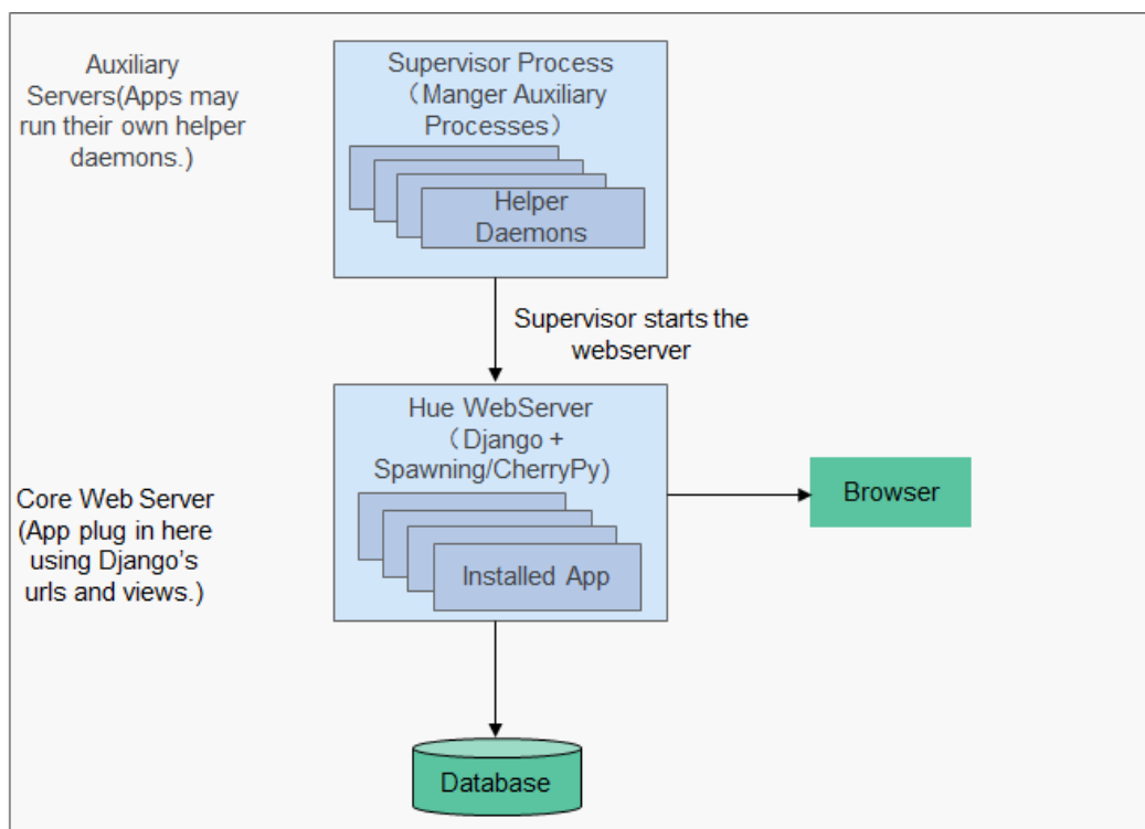
图 1-63 Hue 架构示意图
