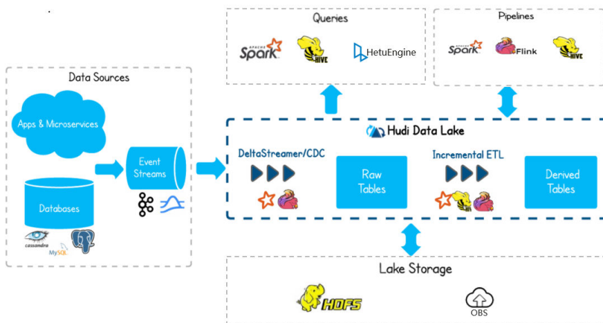
图 1-62 Hudi 基本架构
