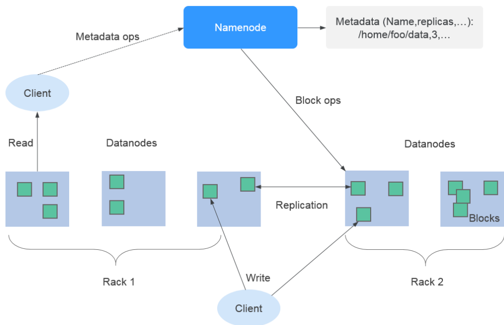
图 1-43 HDFS 架构
