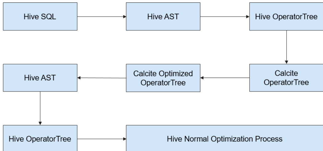
图 1-58 实现流程图
