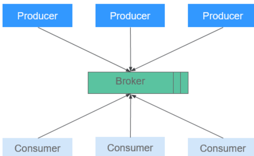
图 1-65 Kafka 结构
