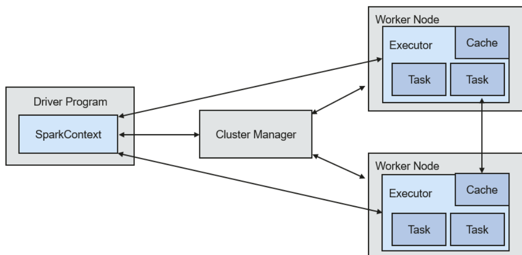
图 1-103 Spark 架构
