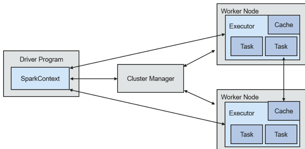
图 1-85 Spark 结构
