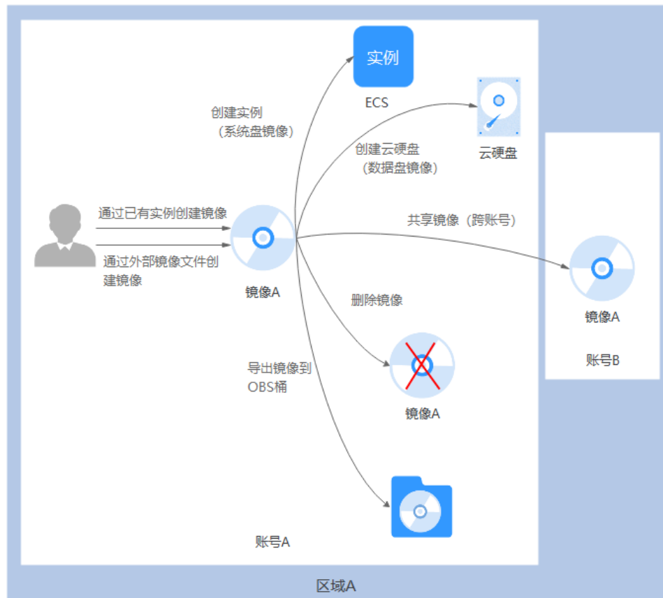
图 1-2 私有镜像生命周期
