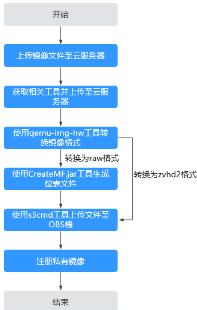
图 3-39 导入流程（基于 Linux 操作系统环境）
