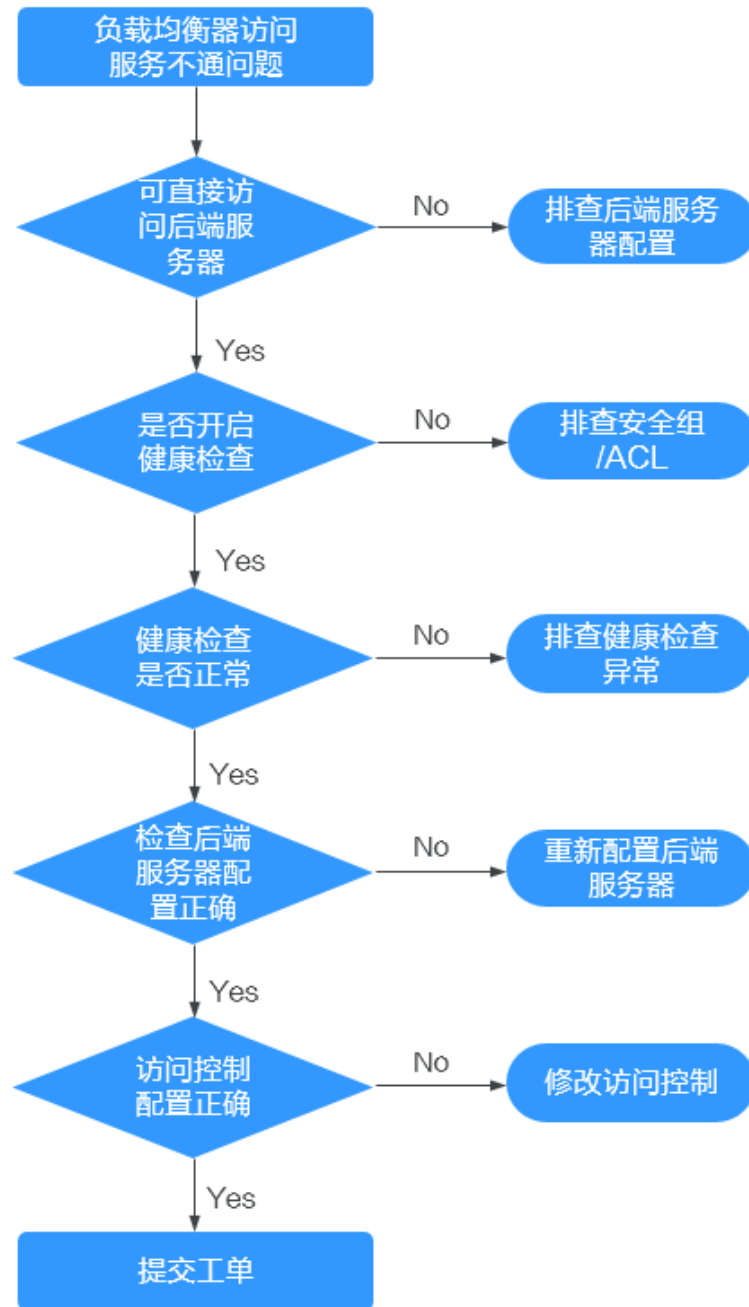
图 18-2 排查思路
