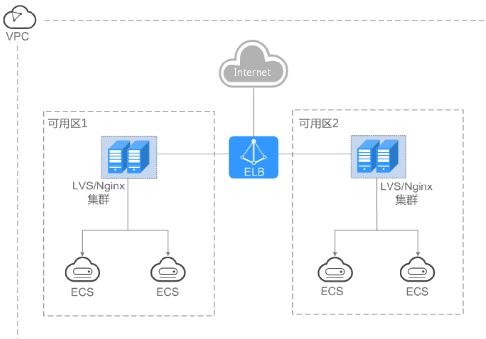
图 1-4 高可用
