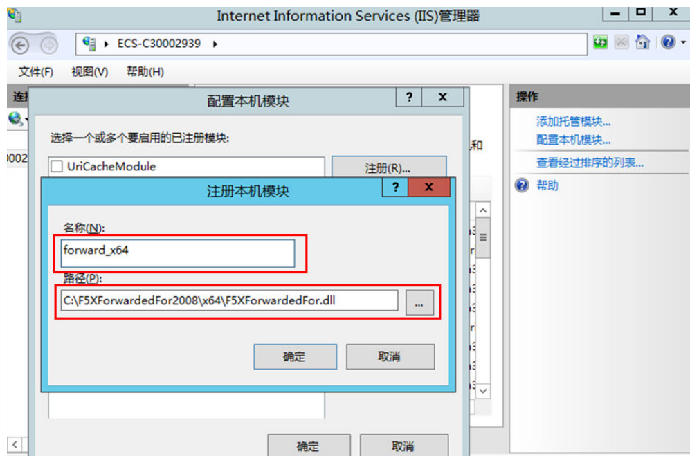
图 18-28 注册插件
