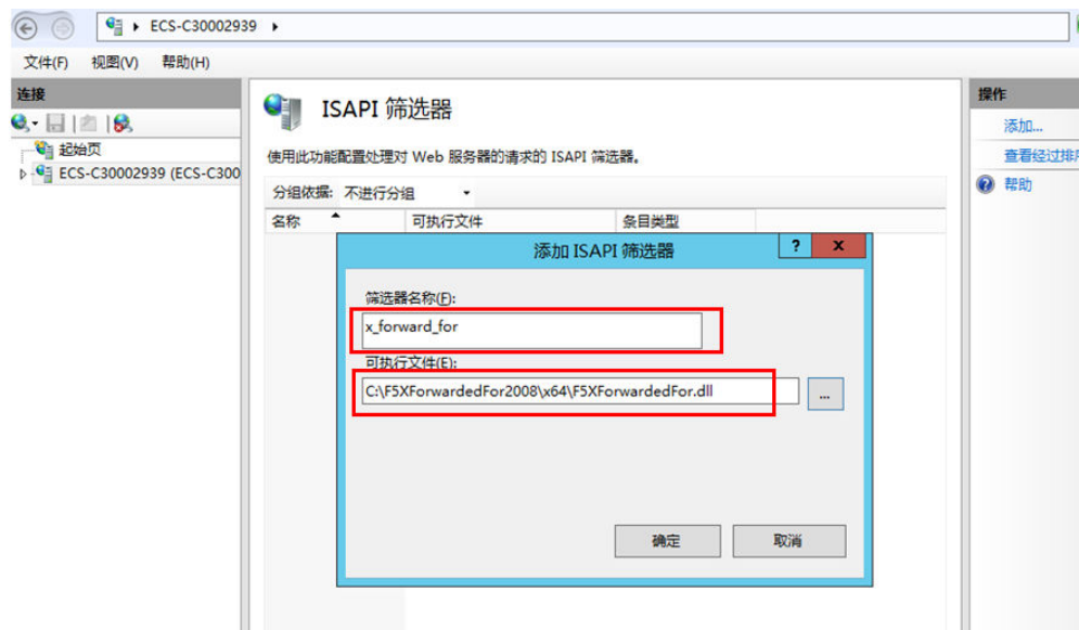
图 18-30 添加授权
