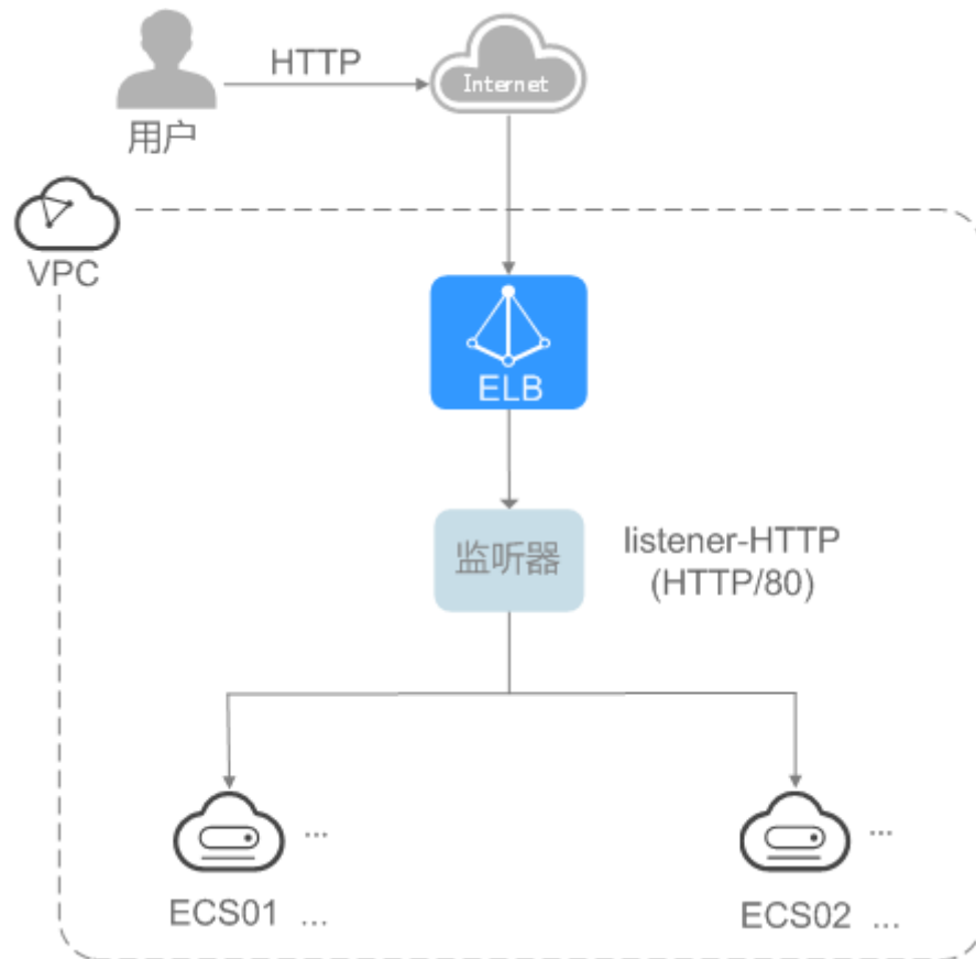
图 2-1 基础版
