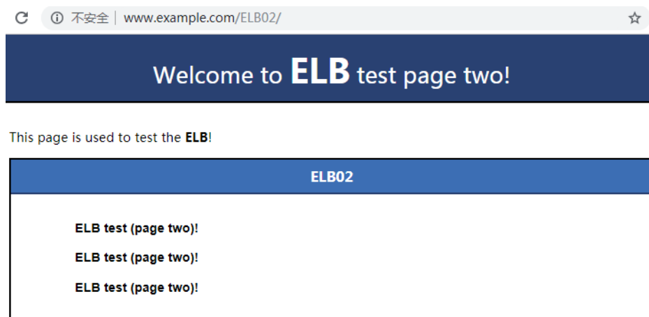
图 2-18 访问到 ECS02
