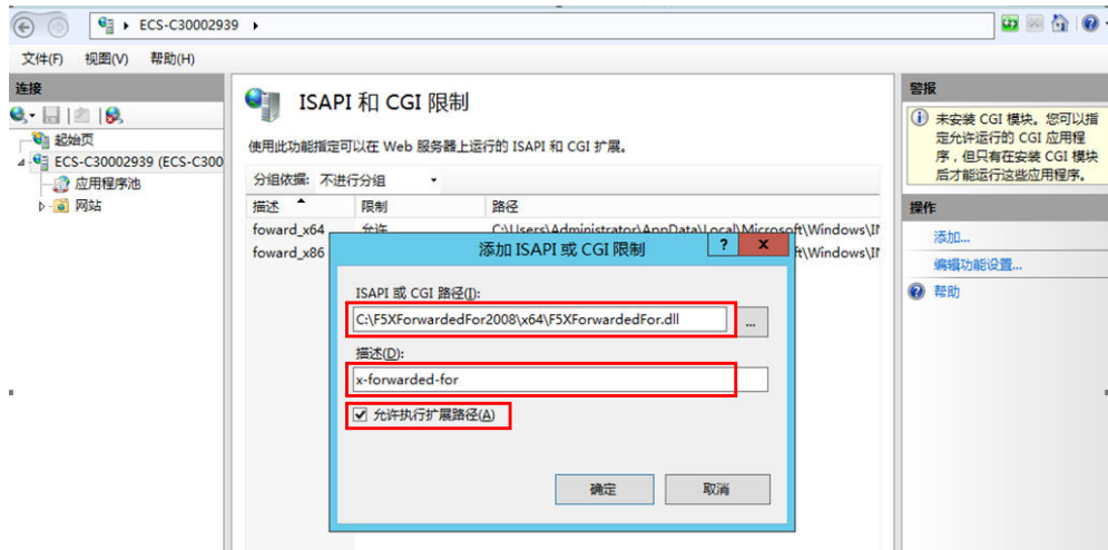
图 18-31 允许执行
