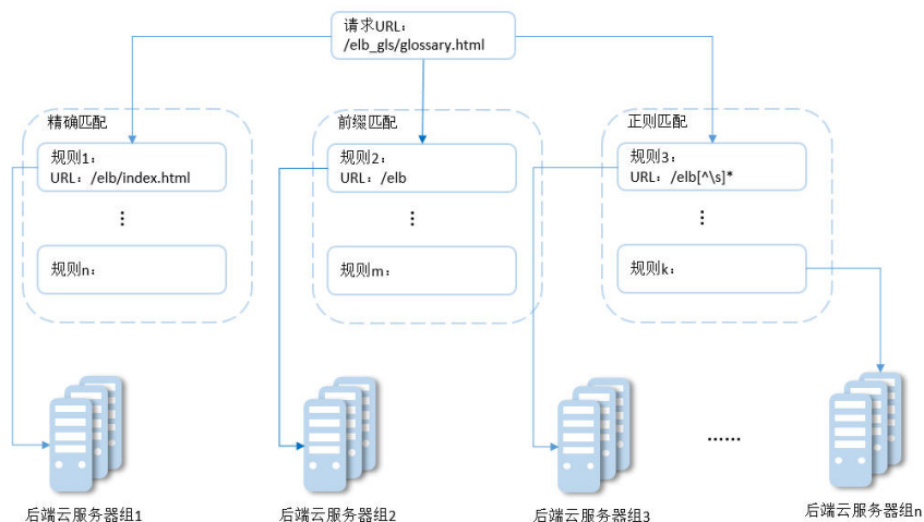
图 5-1 转发示例
