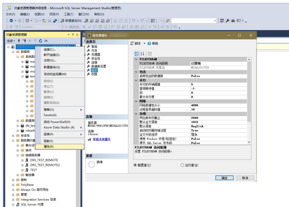
图 5-11 查看本地实例最大并行度值
