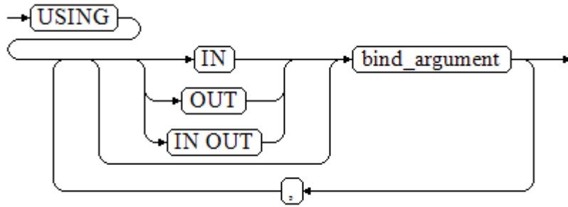
图 13-14 using_clause-4
