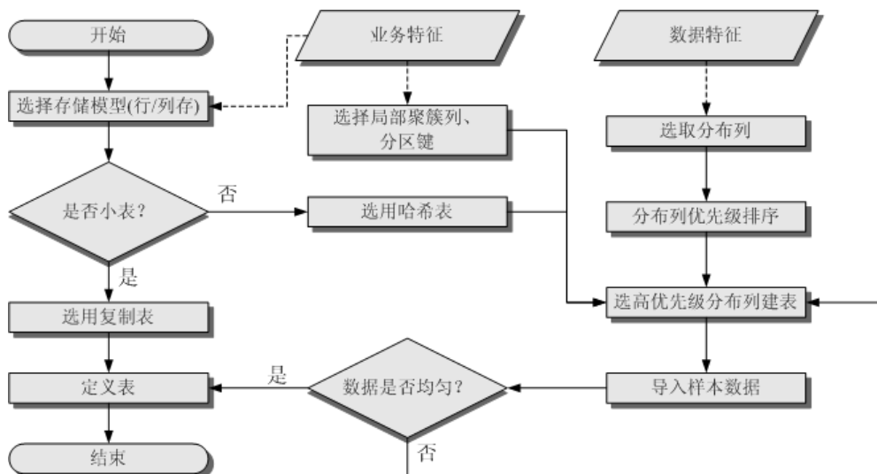
图 11-4 表定义流程
