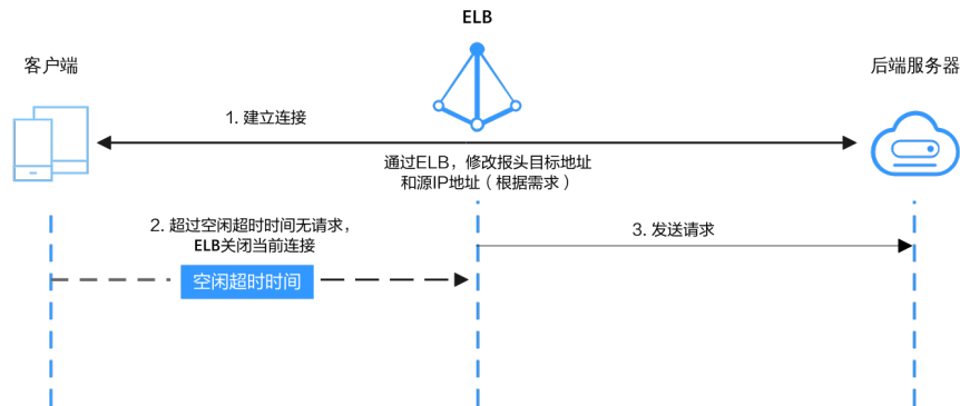
图 6-2 四层监听器超时时间示意图
