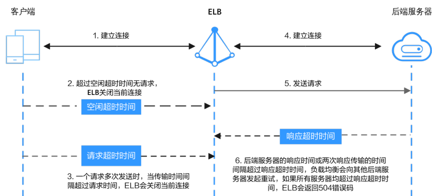
图 6-1 七层监听器超时时间示意图
