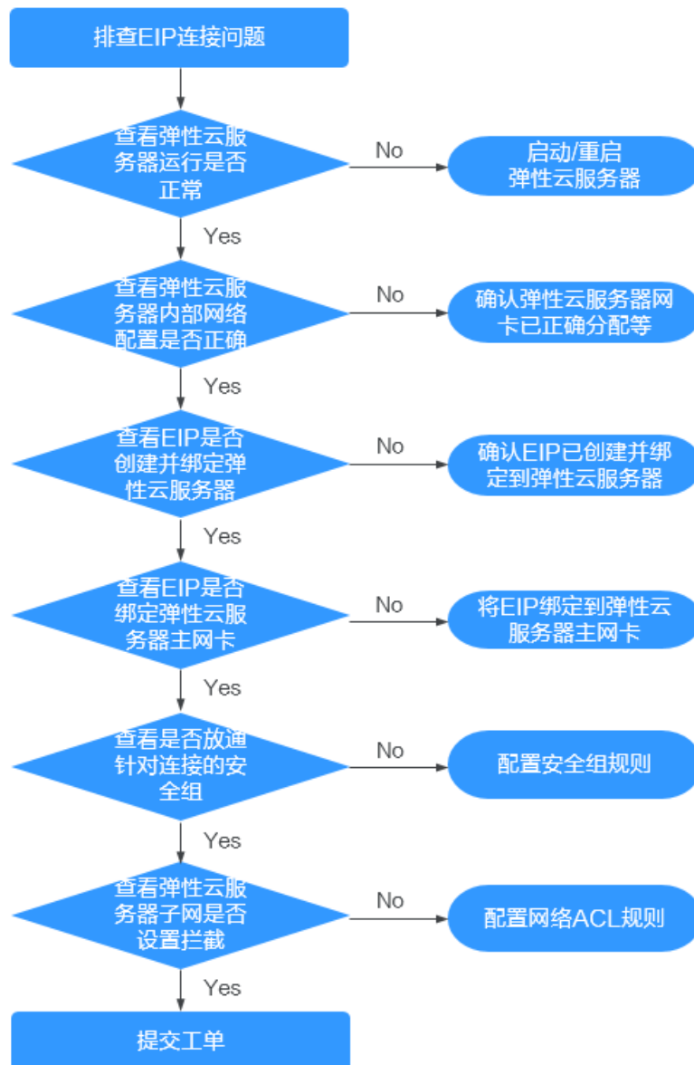
图 5-2 排查思路
