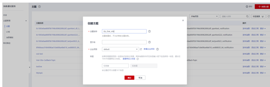
图 6-10 创建主题
