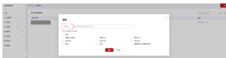
图 6-2 授权
