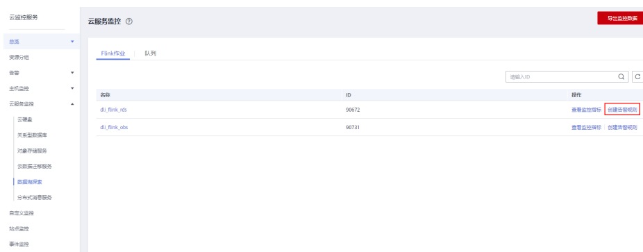
图 6-15 云服务监控
