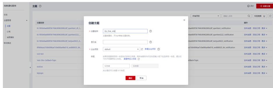
图 6-10 创建主题
