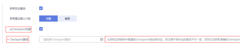
图 6-21 开启 Checkpoint
