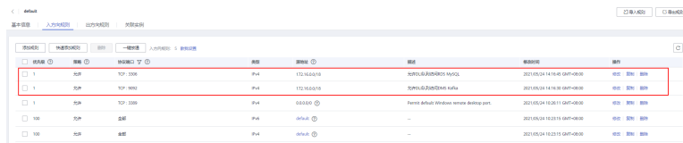
图 4-8 安全组规则
