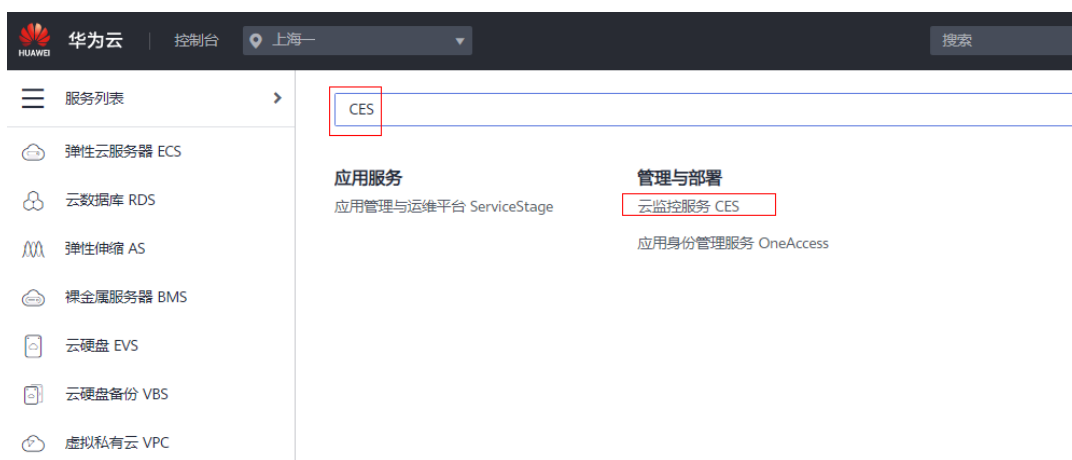
图 2-4 搜索 CES
