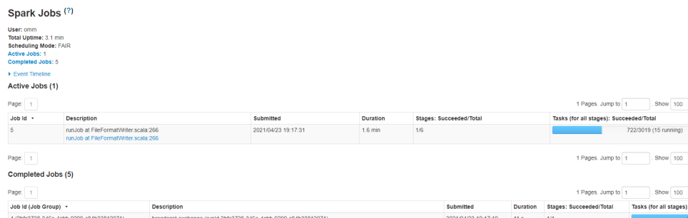
图 7-2 SparkUI
