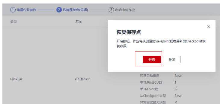
图 6-23 恢复保存点
