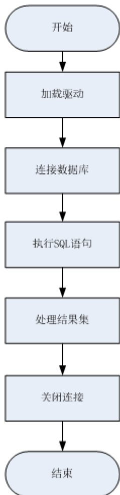
图 6-4 采用 Psycopg2 开发应用程序的流程
