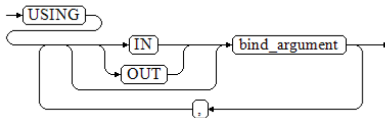
图 13-7 using_clause::=
