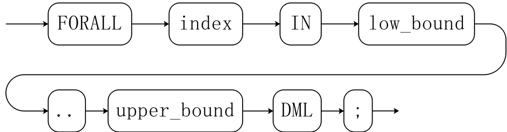
图 13-23 forall::=
