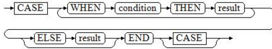
图 12-1 case::=
